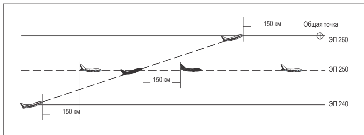
Рис. 5-27А. Интервал 150 км (80 м. миль) между воздушными судами, набирающими высоту, и воздушными судами, находящимися на той же линии пути, при использовании RNAV (см. п. 5.4.2.5.5 c))
