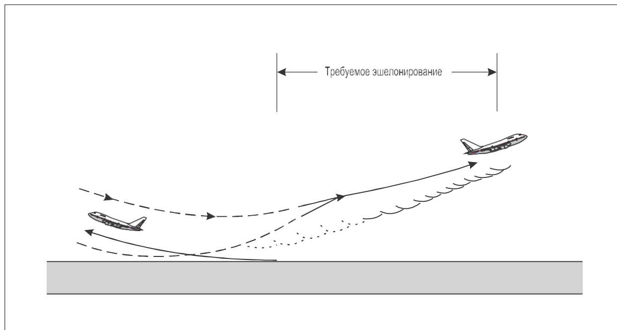
Рис. 5-45. Минимумы эшелонирования при турбулентности в следе при взлетах противоположном направлении (см. пп. 5.8.5.1 а) и 5.8.5.2 а))
