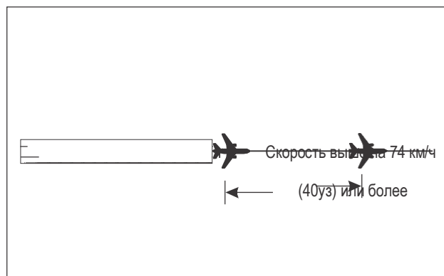
Рис. 5-38. 2-минутный интервал между воздушными судами, следующими по одной и той же линии пути
