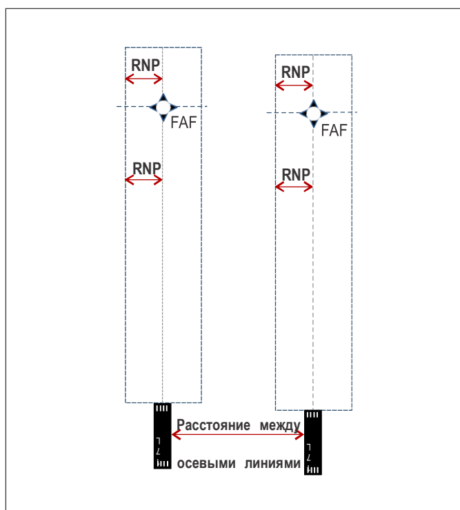
Рис. 6-2. Значение RNP и расстояние между осевыми линиями
