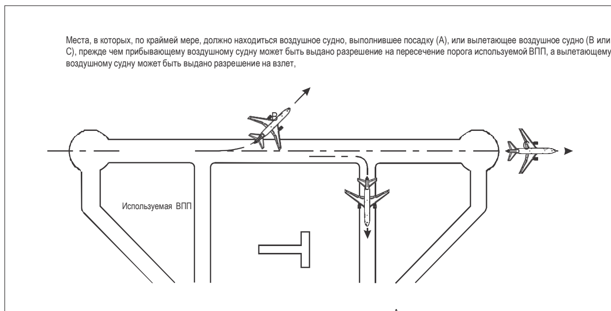
Рис. 7-2. Эшелонирование вылетающих и прибывающих воздушных судов
