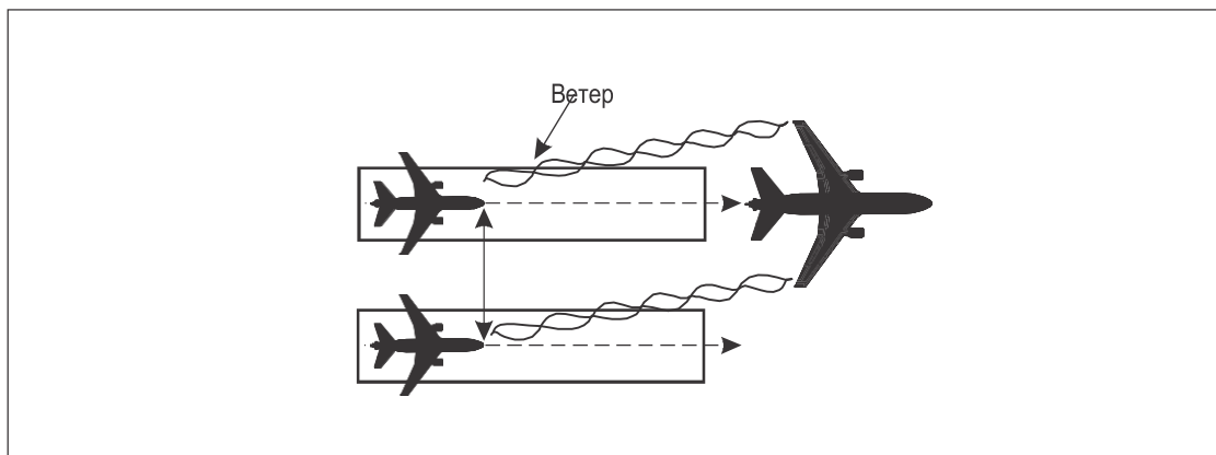
Рис. 5-42. Минимумы эшелонирования при турбулентности в следе для воздушных судов, следующих по той же линии пути (см. пп. 5.8.3.1 а) и б) и 5.8.3.2 а) и б))
