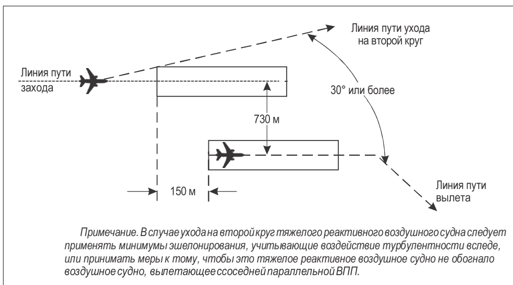
Рис. 6-8. Раздельные параллельные операции на смещенных ВПП (см. п. 6.7.3.6.2)
