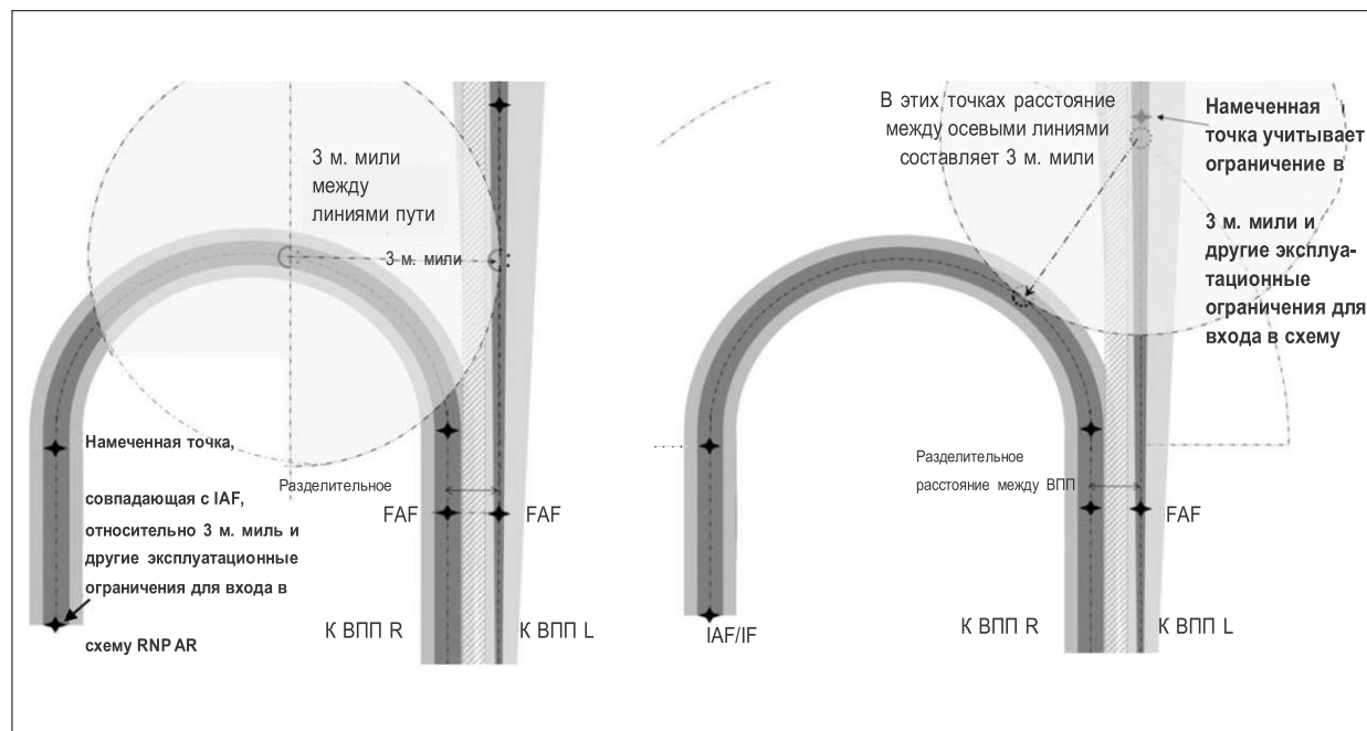
Рис. 6-6. Концепция "воздушного судна, вошедшего в схему RNP AR APCH" (Пример RNP AR APCH/точного захода на посадку с минимумом эшелонирования 3 м. мили)
