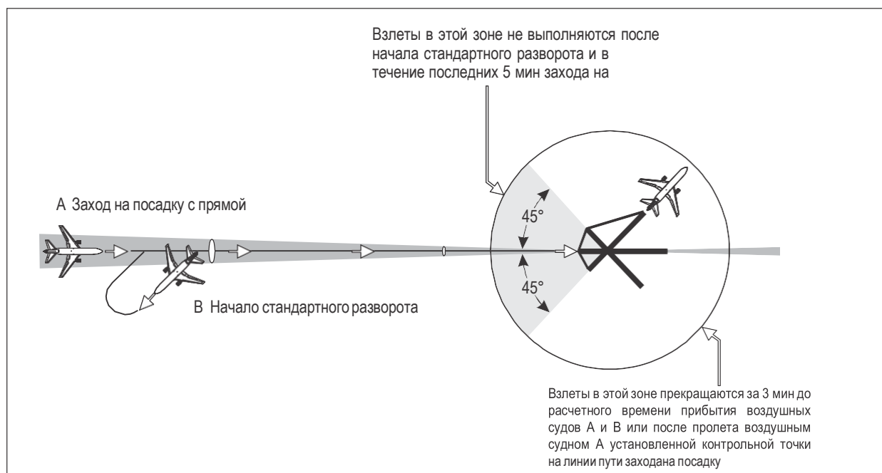
Рис. 5-40. Эшелонирование вылетающих и прибывающих воздушных судов (см. пп. 5.7.1.1 b) и 5.7.1.2 b))
