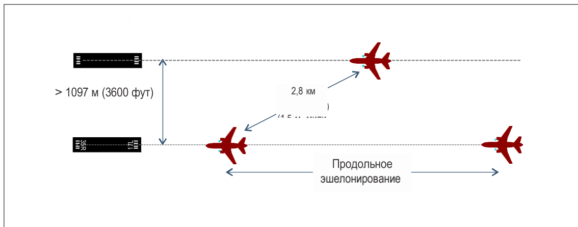
Рис. 6-4. Диагональное эшелонирование для расстояния между осявыми линиями, которое превышает 1097 м (3600 фут), но меньше или равно 2529 м (8300 фут)
