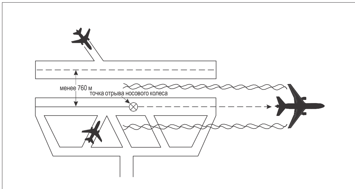
Рис. 5-44. Минимумы эшелонирования при турбулентности в следе для воздушных судов, следующих по той же линии пути (см. пп. 5.8.3.3 и 5.8.3.4)
