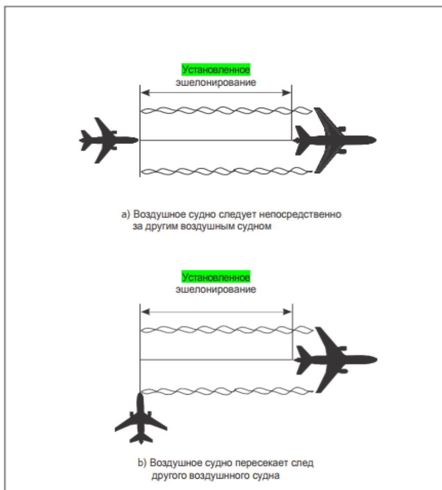
Рис. 8-1. Воздушное судно следует непосредственно за другим воздушным судном или воздушное судно пересекает след другого воздушного судна (см. пп. 8.7.3.4)
