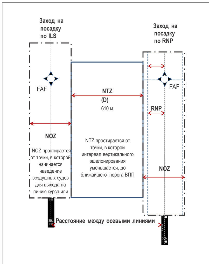
Рис. 6-1 Расстояние между осевыми линиями, NTZ и NOZ
