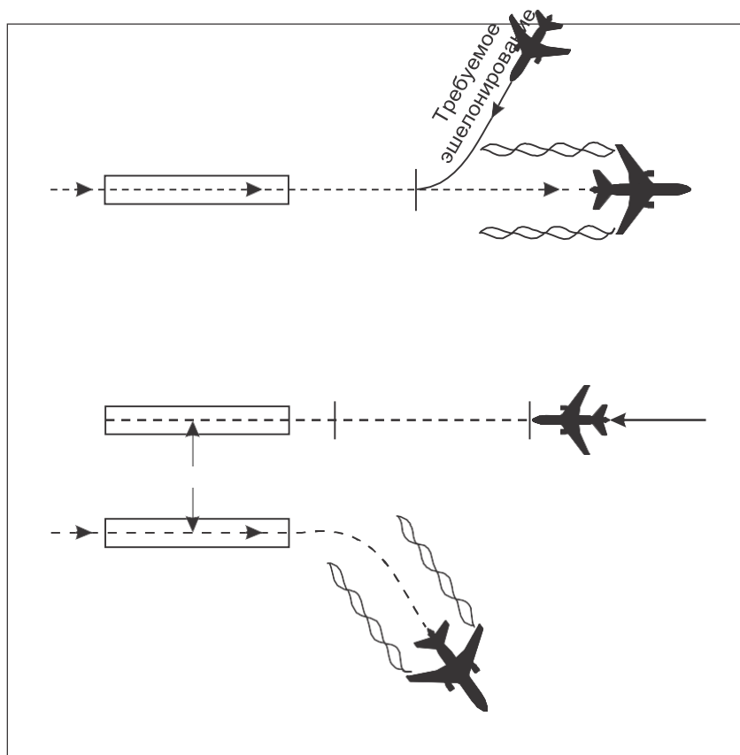
Рис. 5-46. Минимумы эшелонирования при турбулентности в следе при посадке с противоположного направления (см. пп. 5.8.5.1 b) и 5.8.5.2 b))
