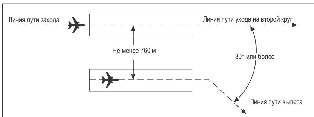
Рис. 6-7. Раздельные параллельные операции (см. п. 6.7.3.6.1 б))
