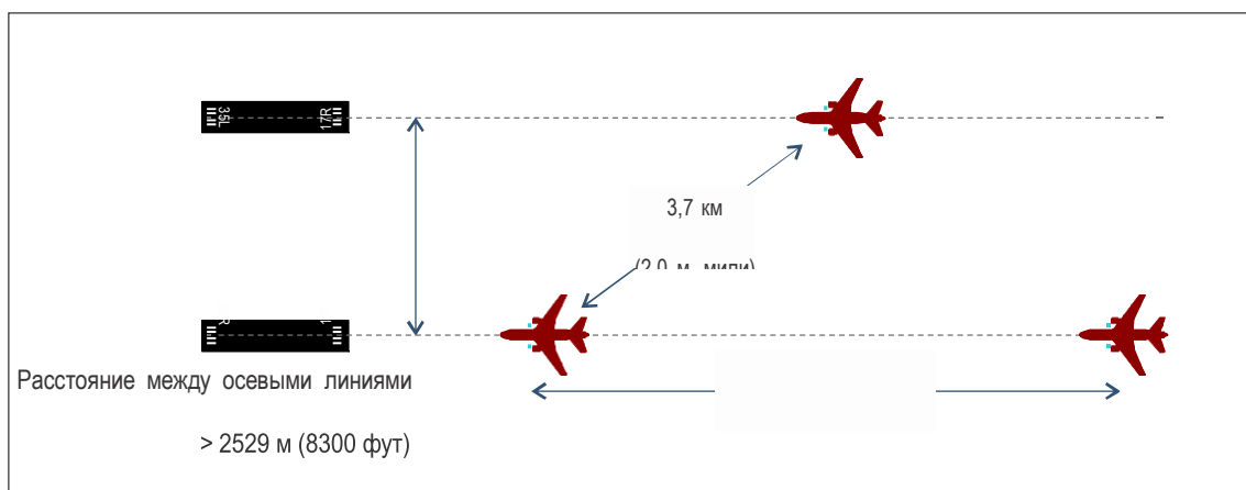
Рис. 6-3. Диагональное эшелонирование для расстояния между осевыми линиями, превышающего 2529 м (8300 фут)
