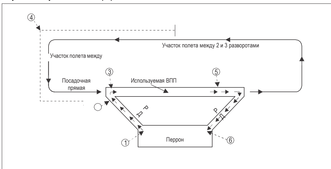
Рис. 7-1. Установленные позиции воздушного судна, видимые с местоположения аэродромного диспетчерского пункта (см. п. 7.6.2)
