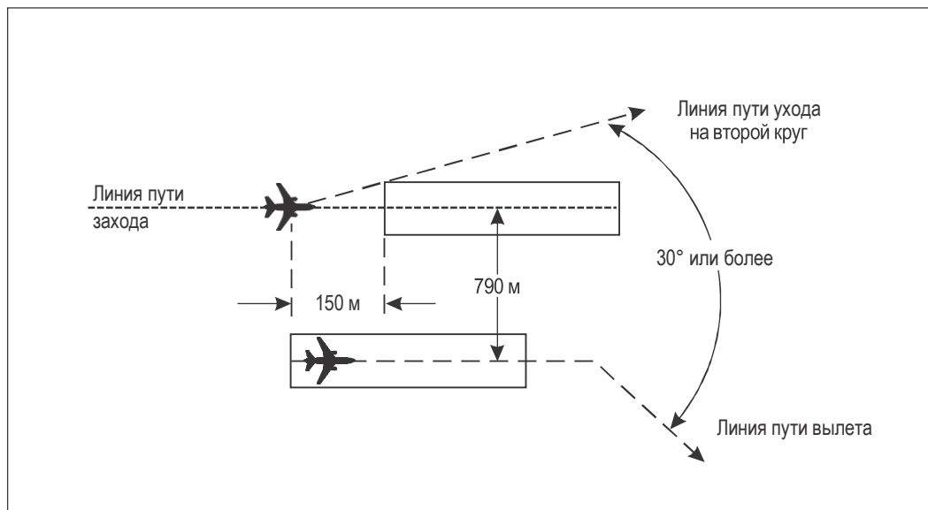
Рис. 6-9. Раздельные параллельные операции на смещенных ВПП (см. п. 6.7.3.6.2)
