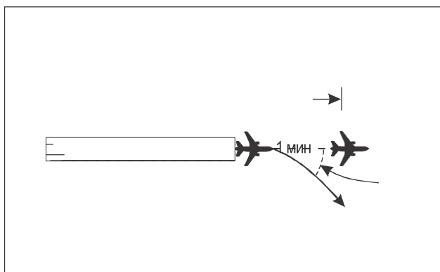
Рис. 5-37. 1-минутный интервал между вылетающими воздушными судами, следующими по линиям пути, расходящимся под углом не менее 45° (см. п. 5.6.1)
