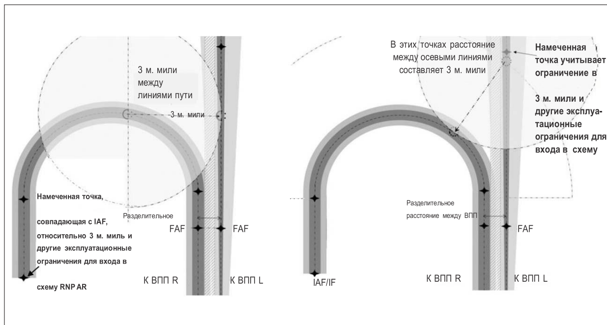
Рис. 6-6. Концепция "воздушного судна, вошедшего в схему RNP AR APCH" (Пример RNP AR APCH/точного захода на посадку с минимумом эшелонирования 3 м. мили)
