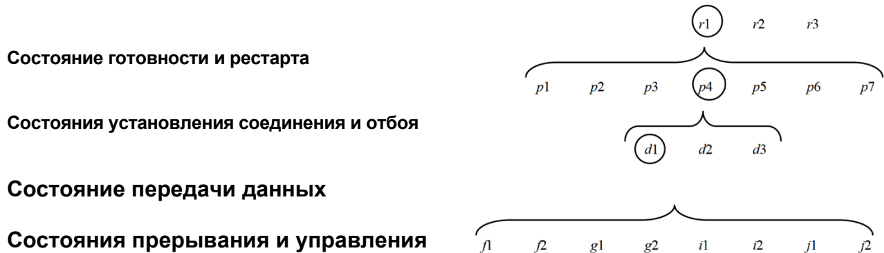
Рис. 5-1. Структура поля SD
