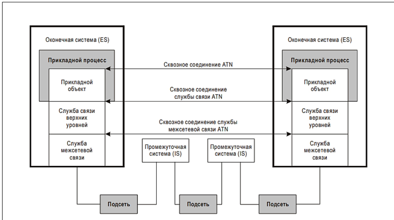
Рис. 3-1. Концептуальная модель ATN
