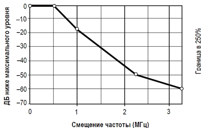
Спектральная маска UAT
