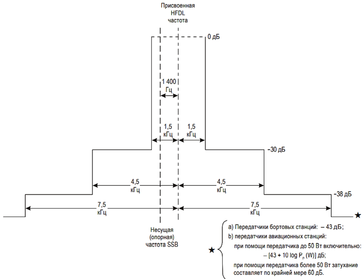
Рис. 11-1. Требуемые пределы спектра (максимальная мощность) для передатчиков
