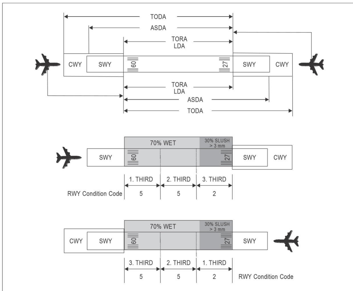
Рис. II-2-1. Сообщение органом ОВД кода состояния ВПП летным экипажам по третям ВПП
