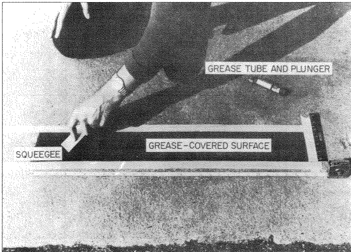
Рис. А2-4. Оборудование, используемое для нанесения консистентной смазки при измерении глубины текстуры поверхности ВПП
