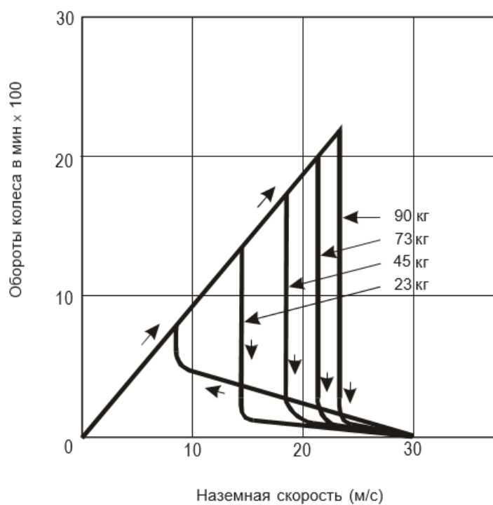
Рис. 2-2. Изменение вращения колеса в зависимости от путевой скорости и нагрузки
