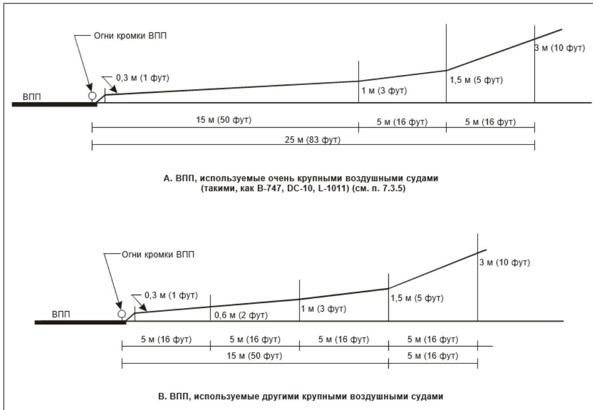
Рис. 7-1. Максимальная высота снежного профиля
