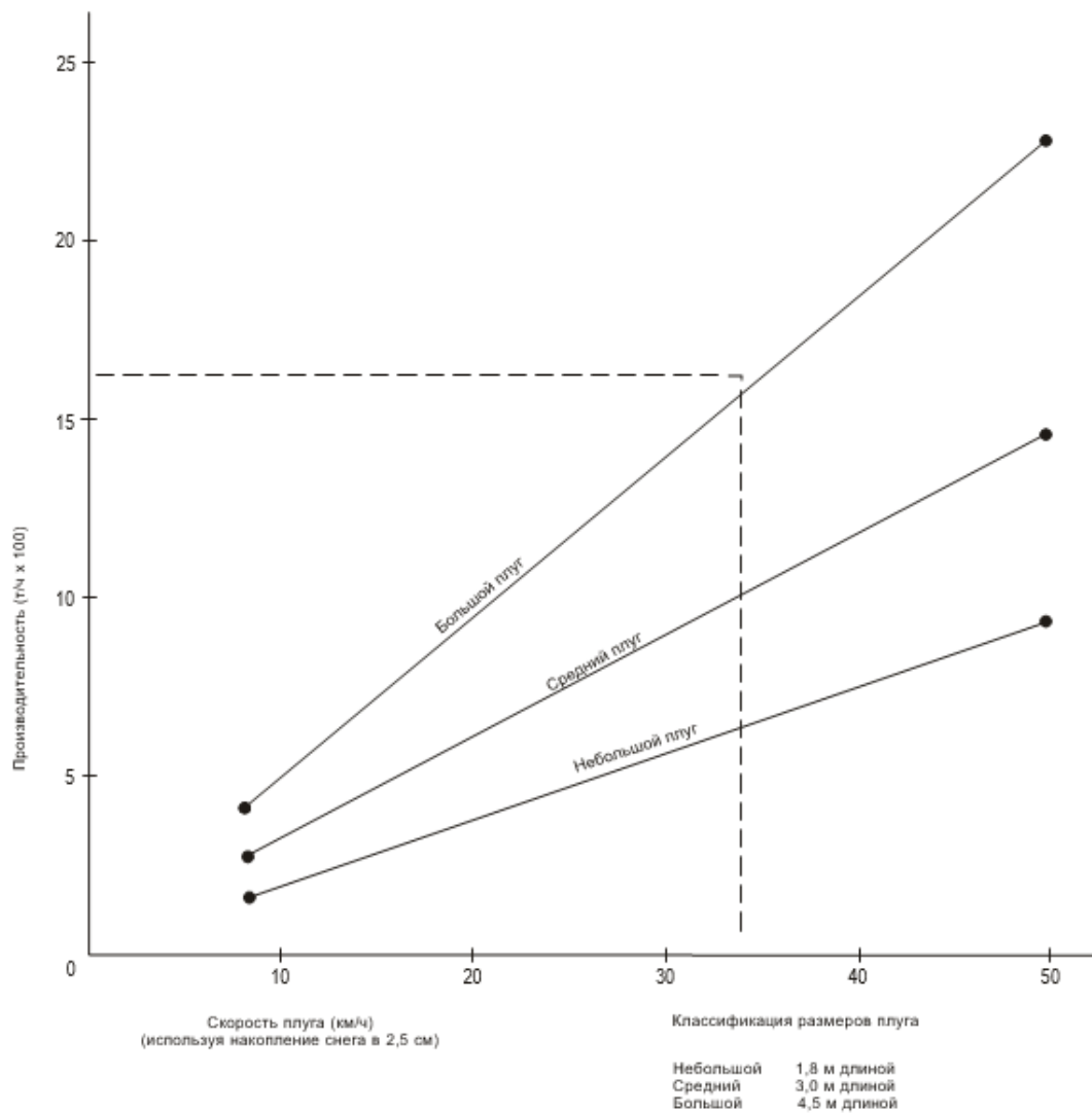
Рис. 7-17. Пример выбора плуга
