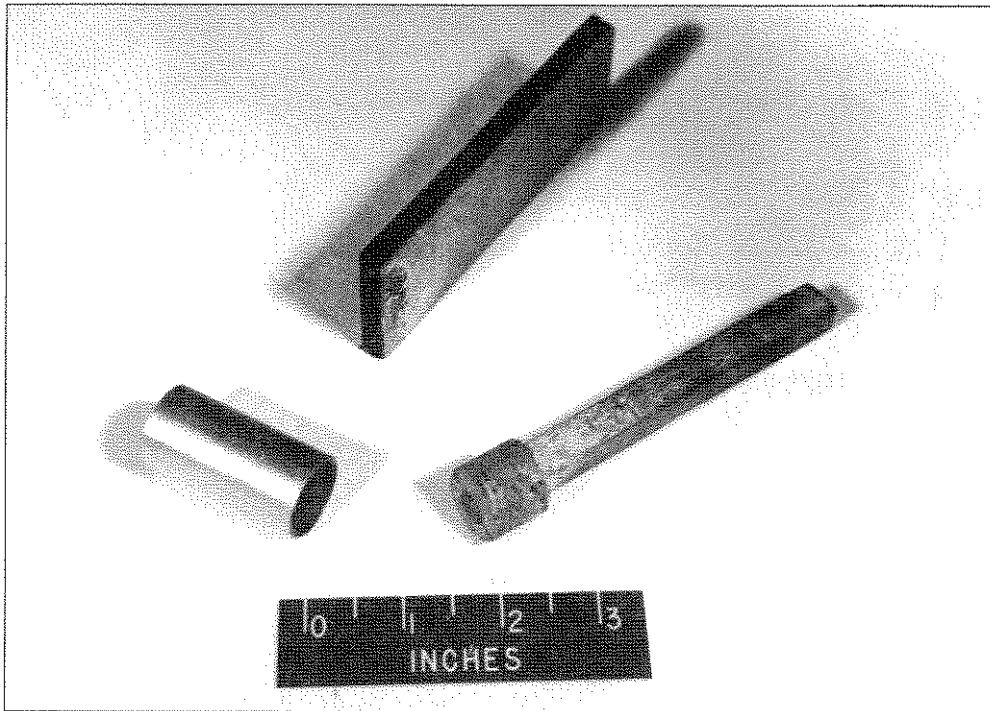
Рис. А2-1. Трубка для измерения объема консистентной смазки, поршень и резиновый отжимной валик
