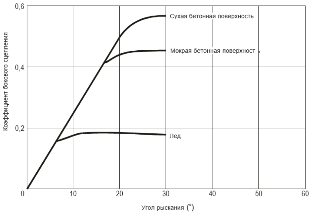
Рис. 1-2. Типичное изменение коэффициента бокового сцепления в зависимости от угла рыскания
