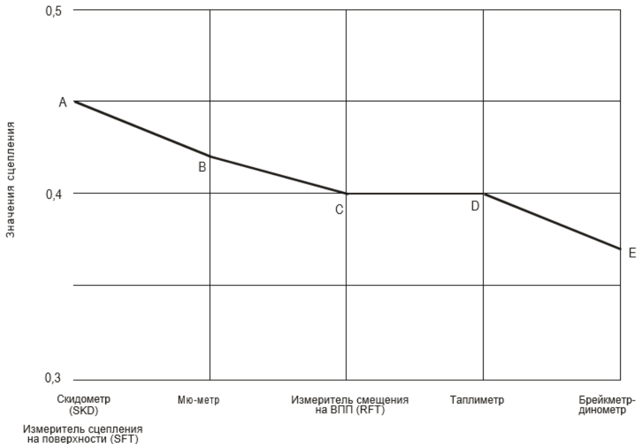
Рис. 5-3. Корреляционный график для устройств измерения сцепления на покрытых уплотненным снегом и/или льдом поверхностях
