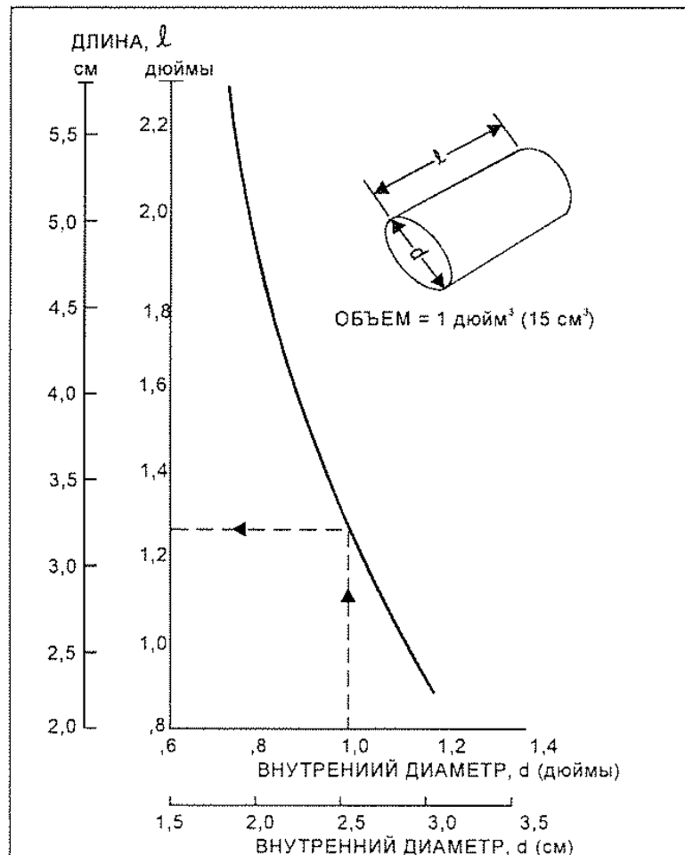
Рис. А2-2. Размеры измерительной трубки для отмеривания одного кубического дюйма, или 15см 3
