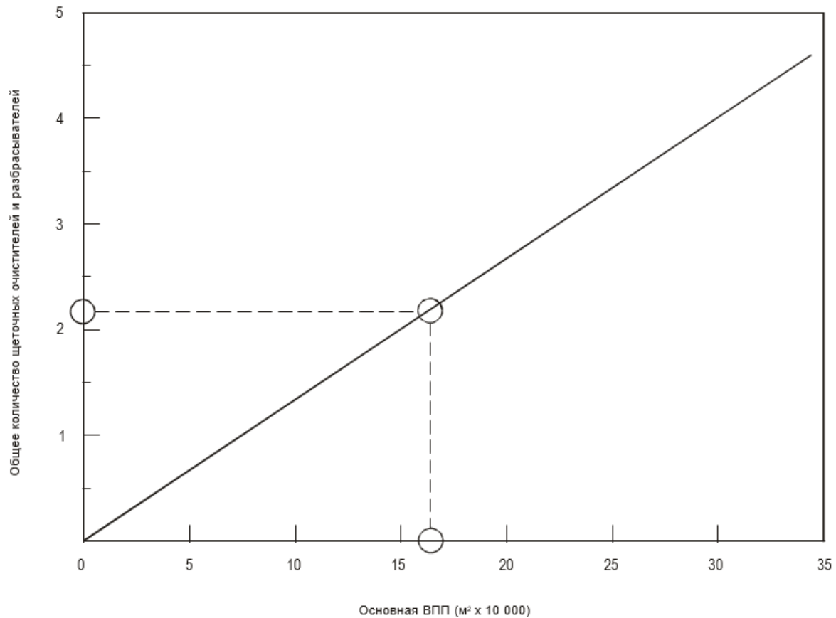
Рис. 7-16. Выбор разбрасывателя/щеточного очистителя
