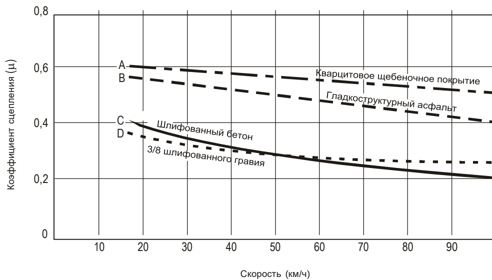
Рис. 1-4. Связь между коэффициентами сцепления при торможении, достигаемого при антиюзном торможении на поверхностях различной текстуры при определенных условиях эксплуатации
