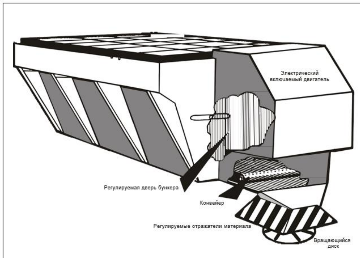
Рис. 7-6. Разбрасыватель песка
