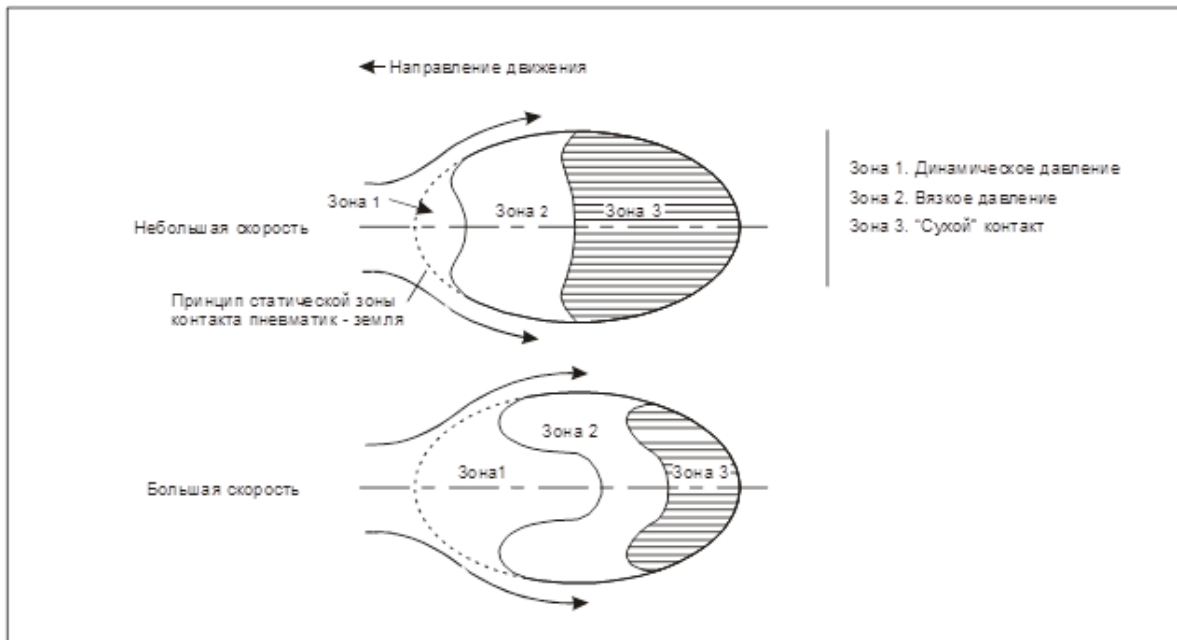
Рис. 1-3. Зоны раздела пневматика с поверхностью
