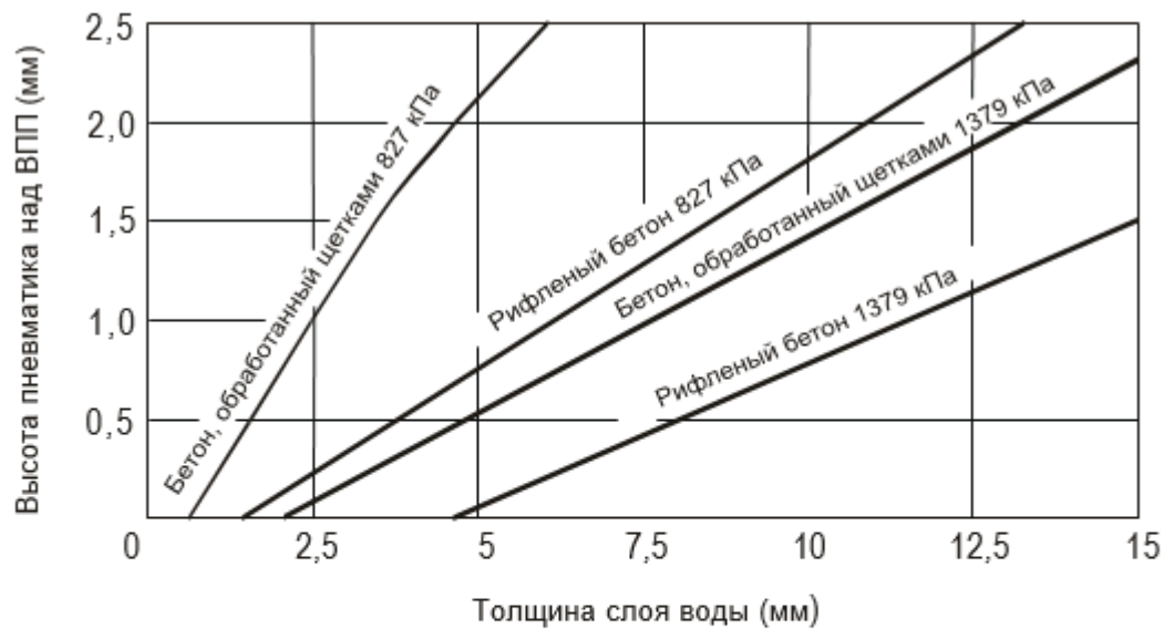
Рис. 2-3. Высота пневматика над ВПП при различных толщине слоя воды, текстуре поверхности и давлении в пневматике при скорости, превышающей скорость глиссирования
