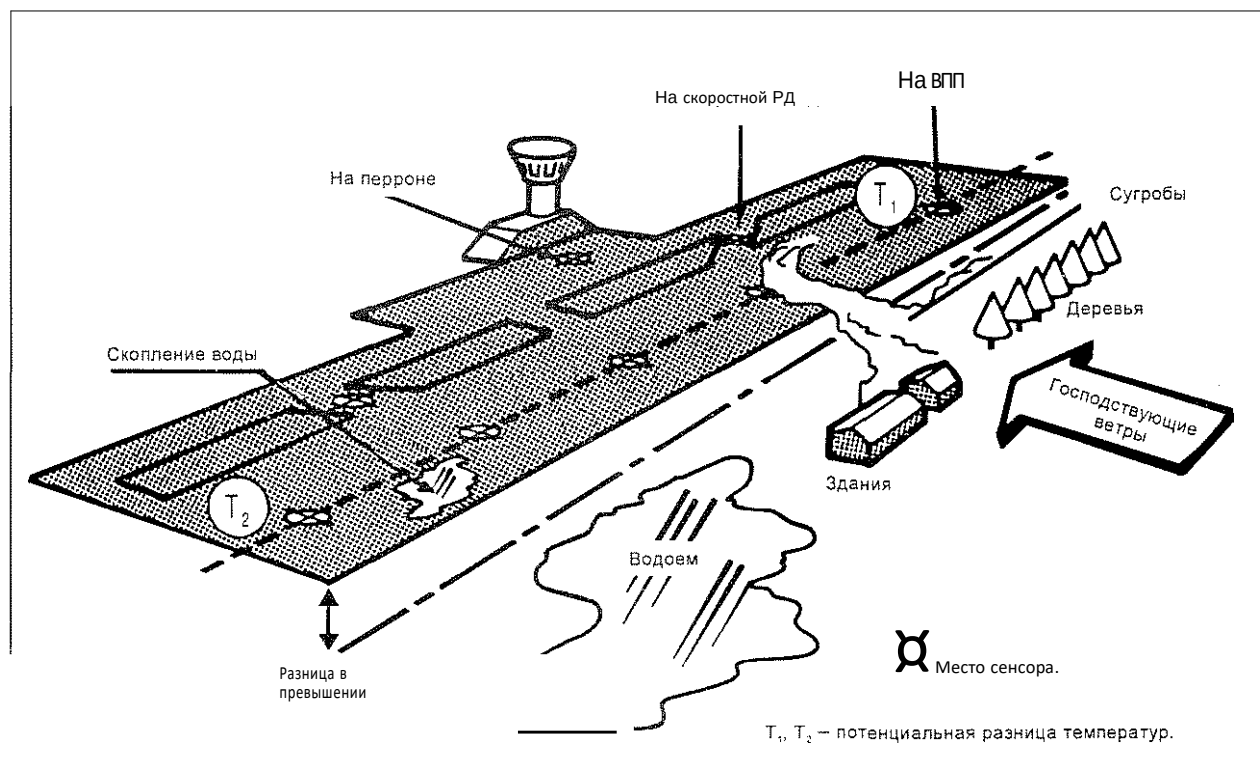
Рис. 7-13. Факторы влияющие на выбор места для датчиков
