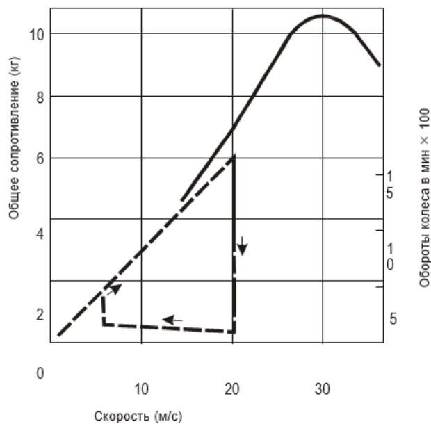
Рис. 2-1. Изменение общего сопротивления небольшого пневматика в зависимости от количества оборотов колеса в минуту и скорости
