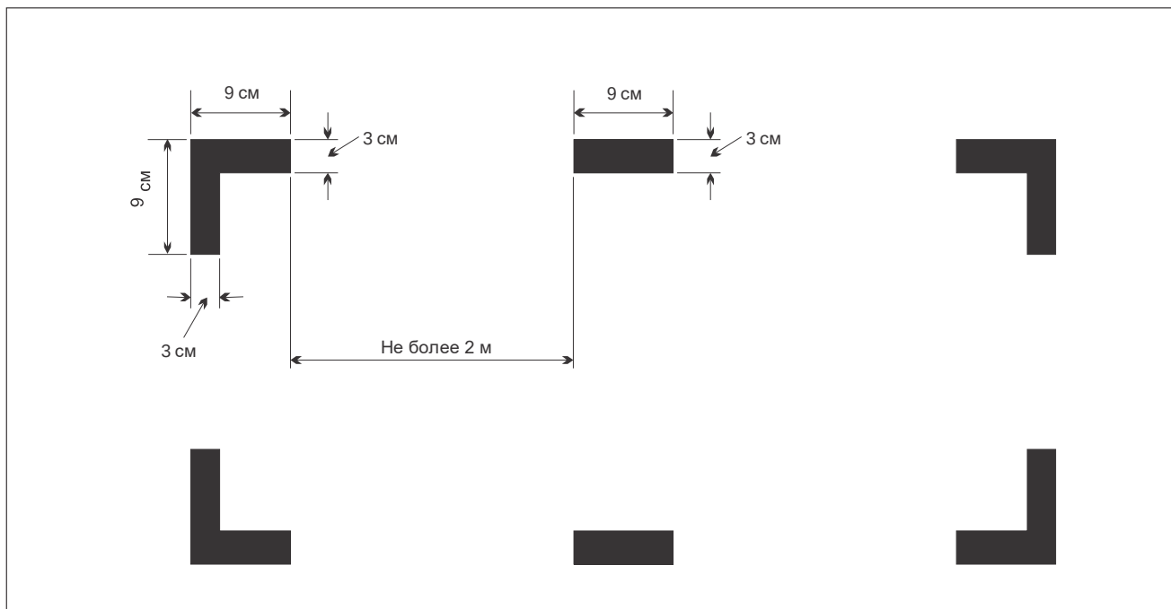
МАРКИРОВКА МЕСТ АВАРИЙНОГО ВСКРЫТИЯ ФЮЗЕЛЯЖА (см. п. 4.2.4)
