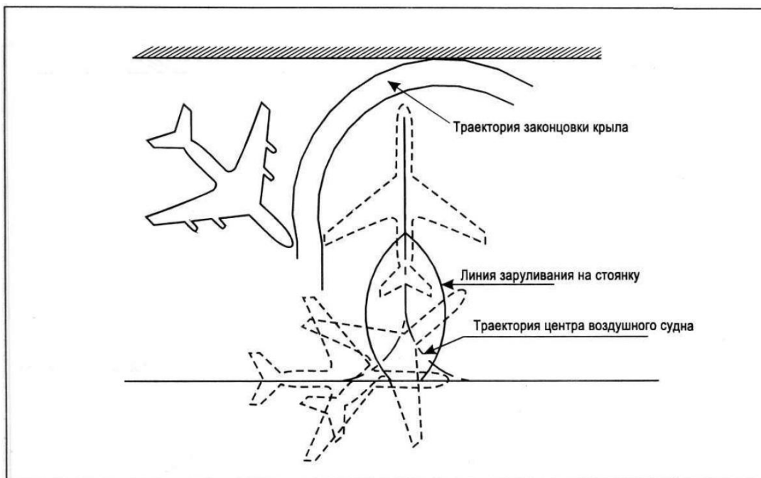
Рисунок 2-2. Простая линия за руливания на стоянку, по которой следует носовое колесо воздушного судна
