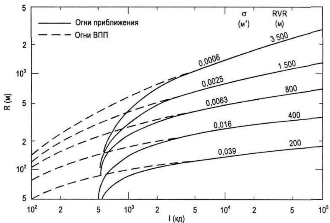
Рисунок А4-2. Дальность видимости R в зависимости от силы света огней I при яркости фона L = 10\,000 кд/м²
