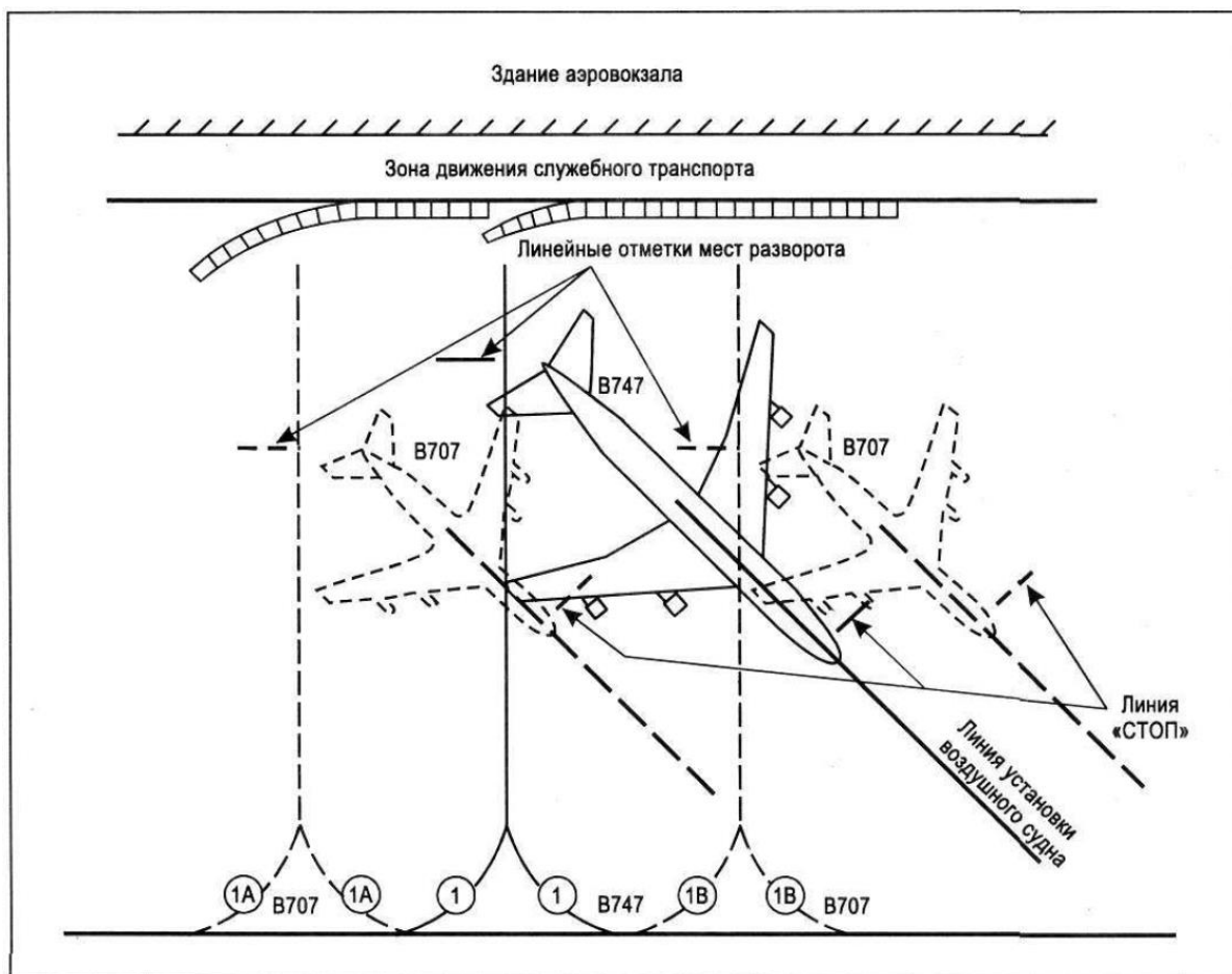
Рисунок 2-8. Один из методов маркировки многоцелевых стоянок
