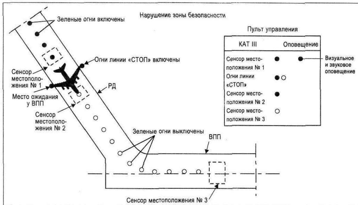
Рисунок 10-6. Управление огнями линии «СТОП» посредством сенсоров местоположения.
