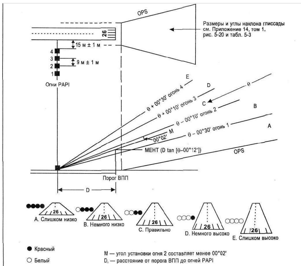
Рисунок 8-6. Размещение огней RAPI и результирующие схемы отображения
