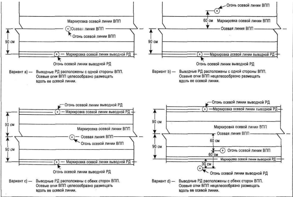
Рисунок 9-2. Маркировка и огни пересечений ВПП и РД
