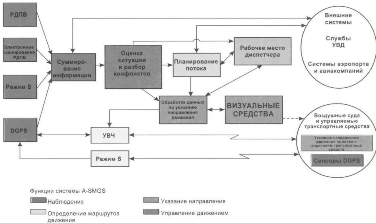
Рисунок 10-1. Пример структурной схемы системы A-SMGCS
