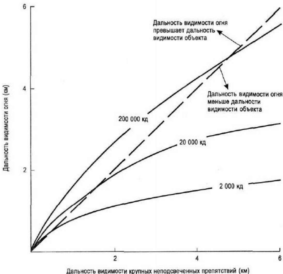
Рисунок 14-1. Сравнение типовых характеристик дальности видимости огней в дневное время и дальности видимости крупных неподсвеченных объектов для трех значений интенсивности огня
