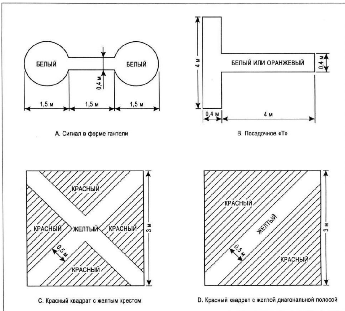
Рисунок 3-1. Сигнальные знаки и посадочное «Т»
