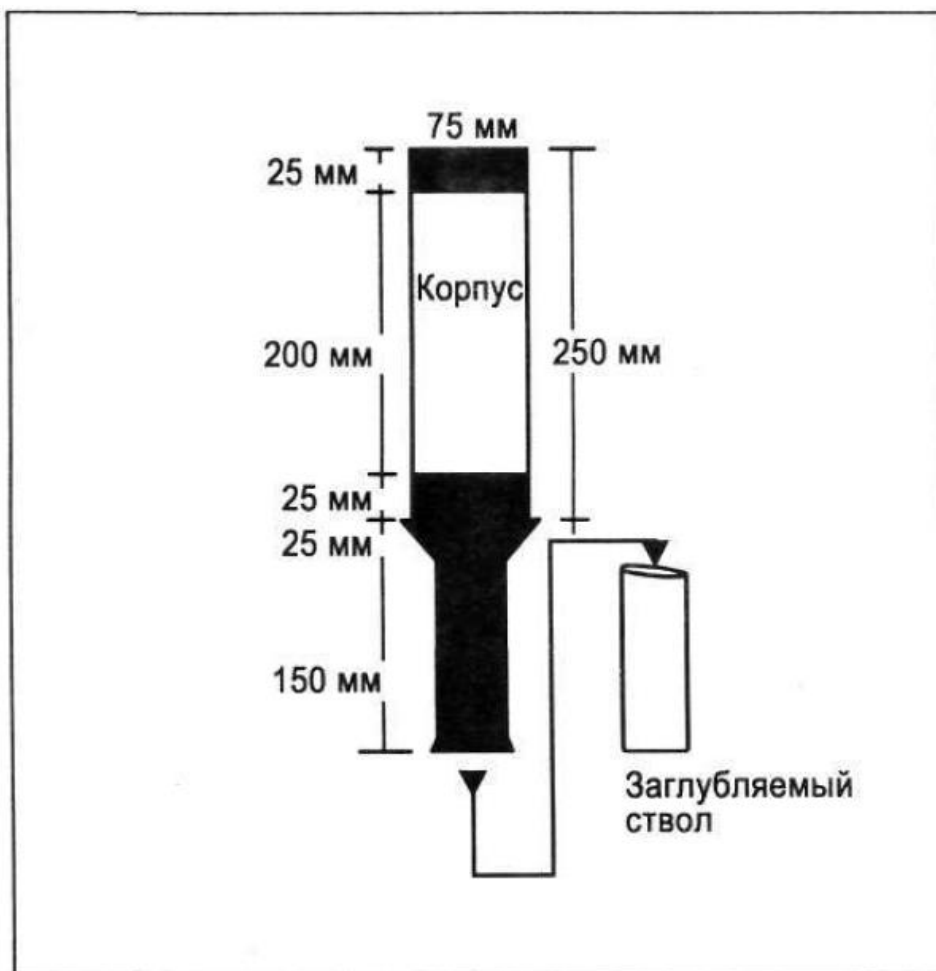
Рисунок 2-10. Маркер кромки РД
