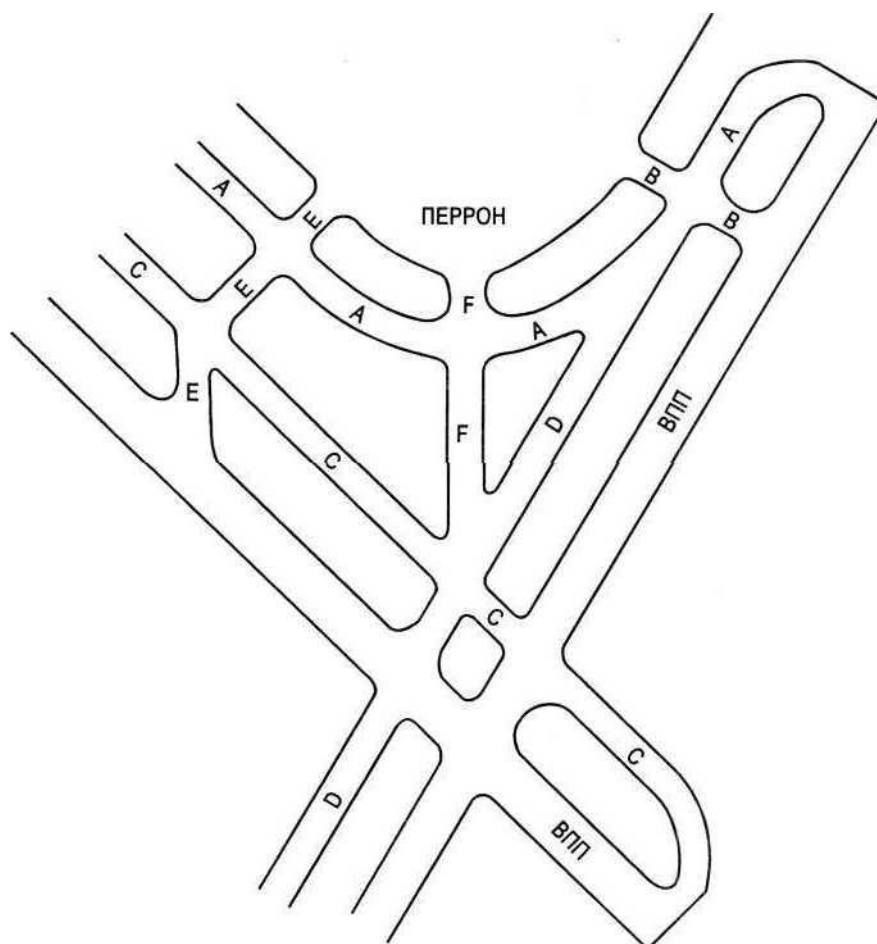
Рисунок 11-6. Буквенные обозначения рулевых дорожек
