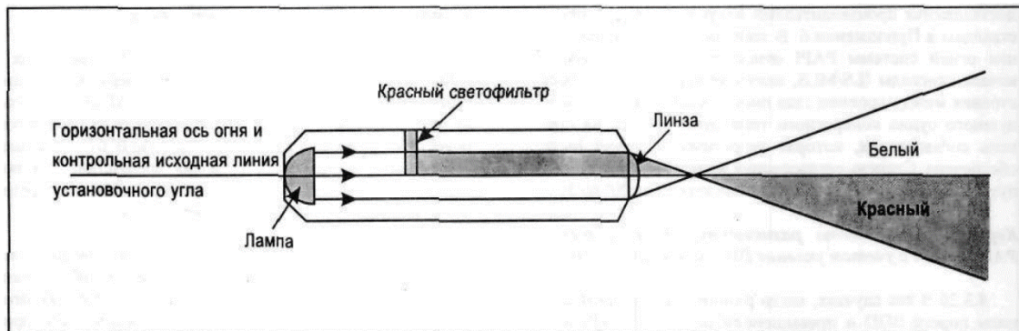
Рисунок 8-9. Огонь системы PAPI
