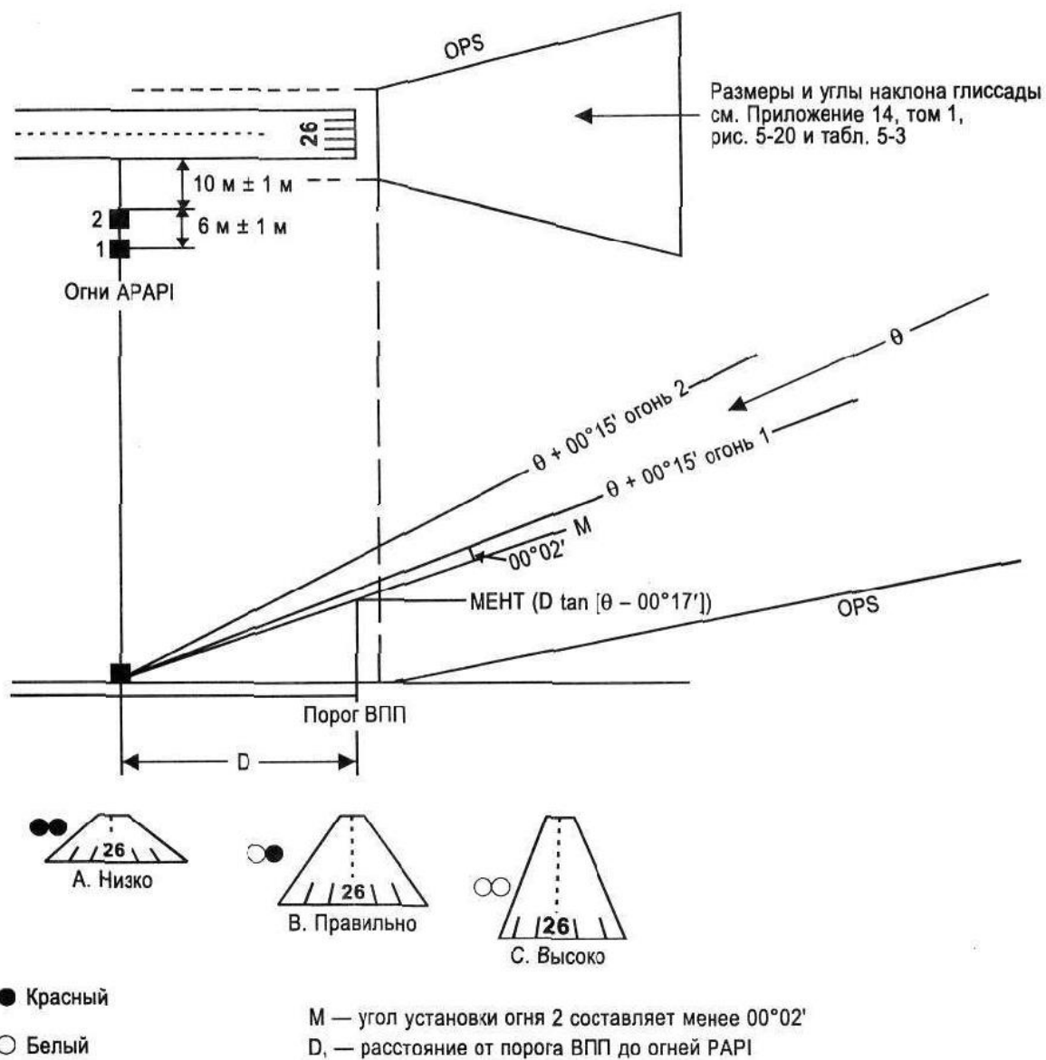
Рисунок 8-7. Размещение огней АРАРІ и результирующие схемы отображения
