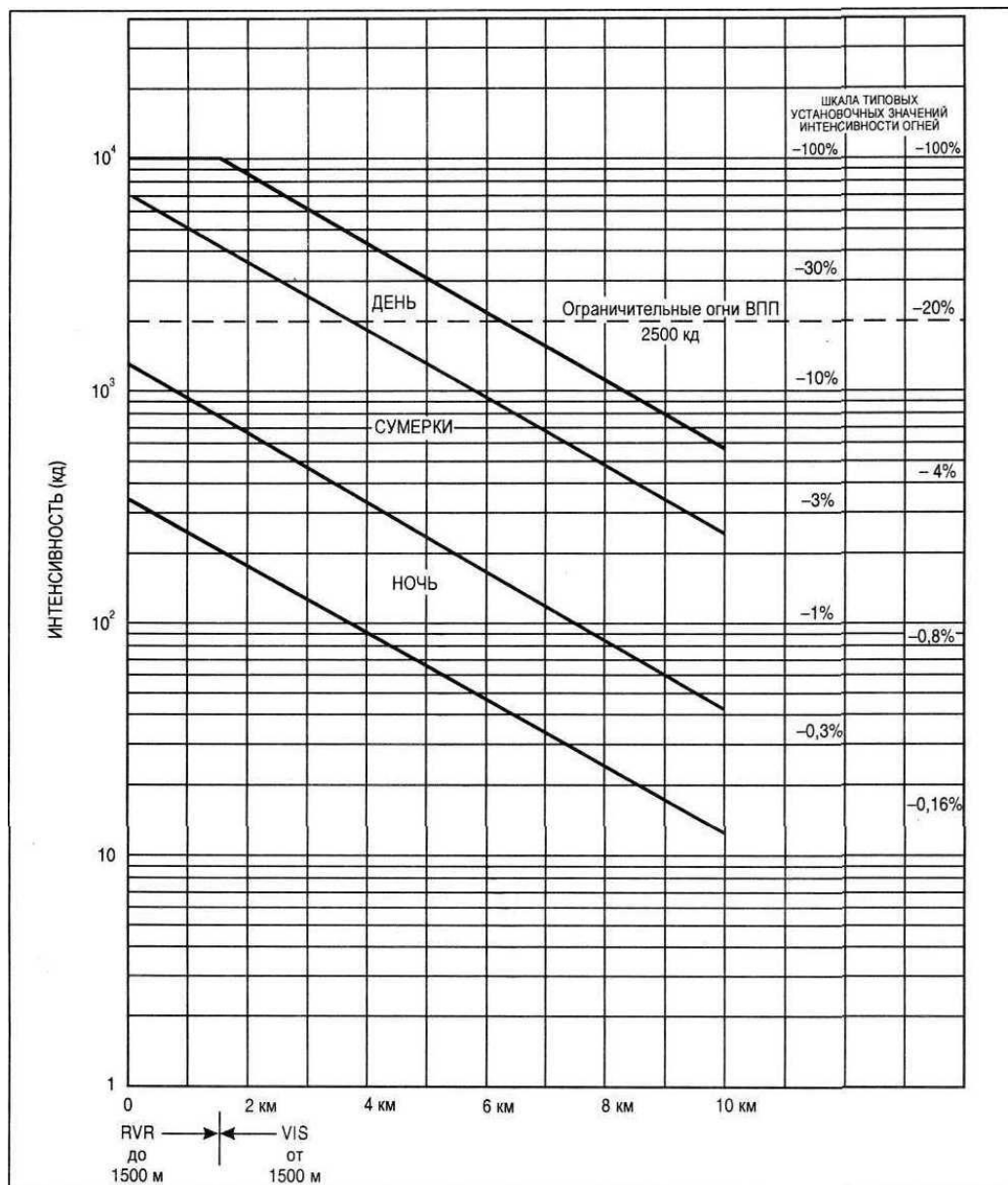
Рисунок 5-2. Боковой ряд огней приближения, огни зоны приземления, осевые огни ВПП
