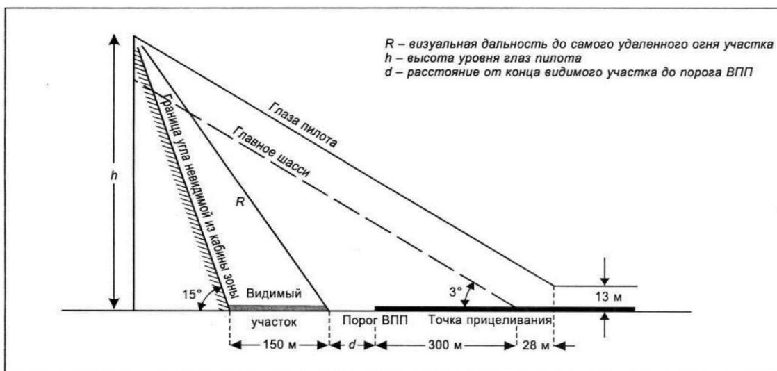
Рисунок A4-1. Геометрические размеры на конечном участке захода на посадку
