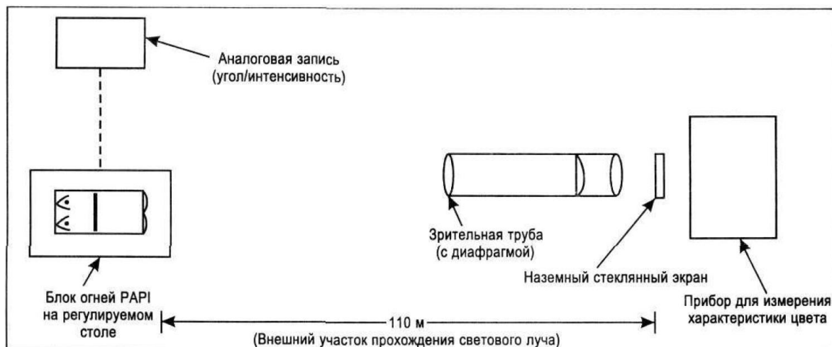
Рисунок 8-10. Схема испытательной лаборатории
