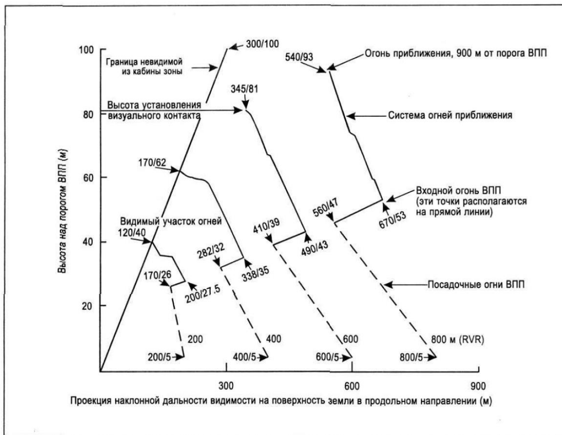
Рисунок А4-3. Пример расчета длины видимого участка системы огней, обеспечиваемого выбором потребных значений силы света (при среднем градиенте тумана)
