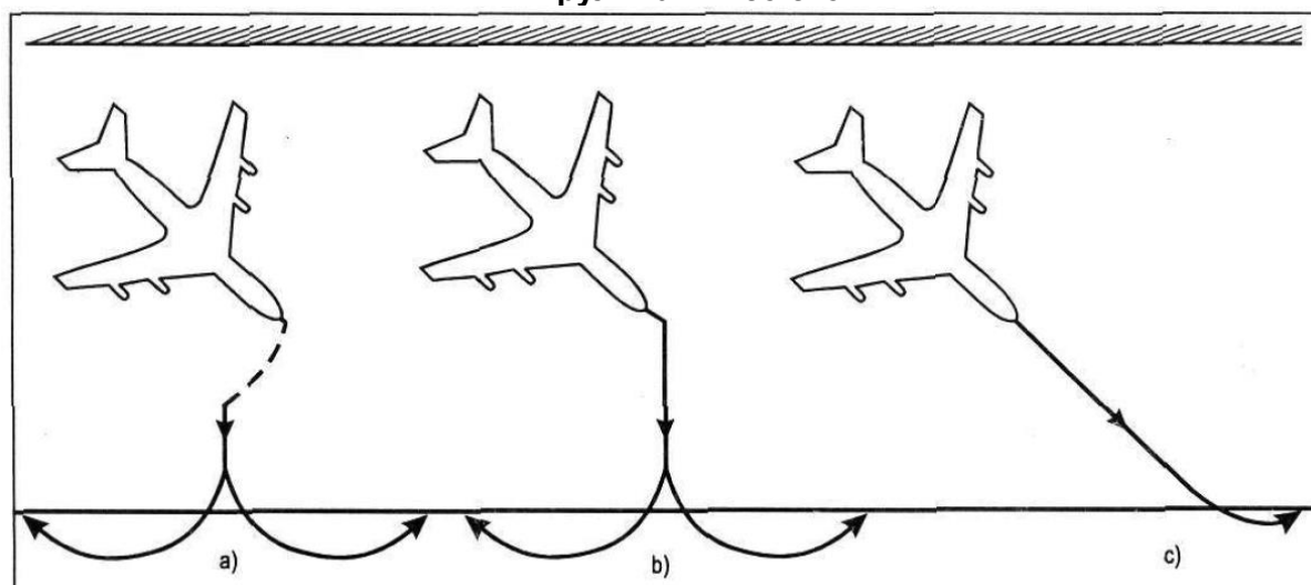
Рисунок 2-6. Обычные линии следования носового колеса воздушного судна при выруливании со стоянки
