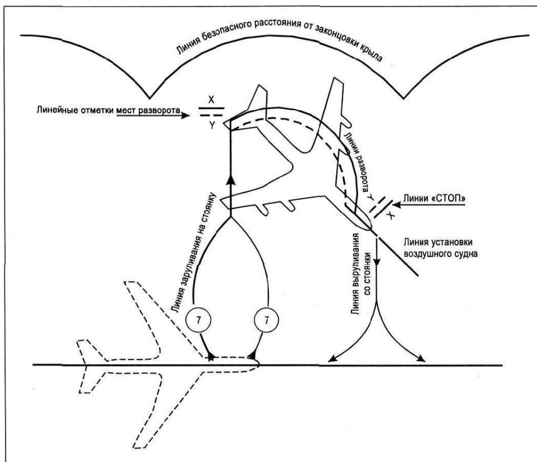
Рисунок 2-9. Образцы контрольных отметок 1
