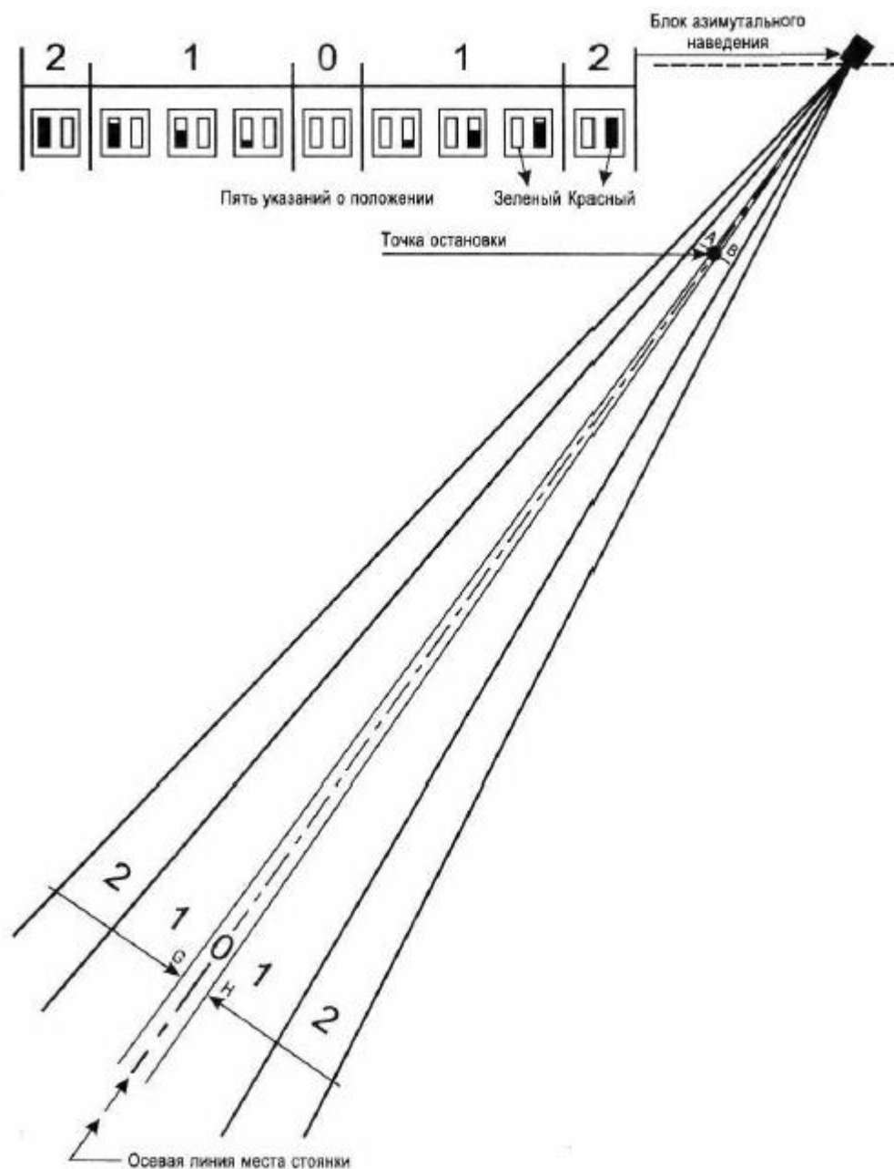
Рисунок 12-3. Блок азимутального наведения системы управления визуальной стыковкой воздушного судна с телескопическим трапом, в которой используются огни
