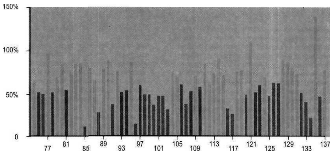
Рисунок 17-1. Освещенность ВПП для операций по категории III до проведения дифференцированного обслуживания огней
