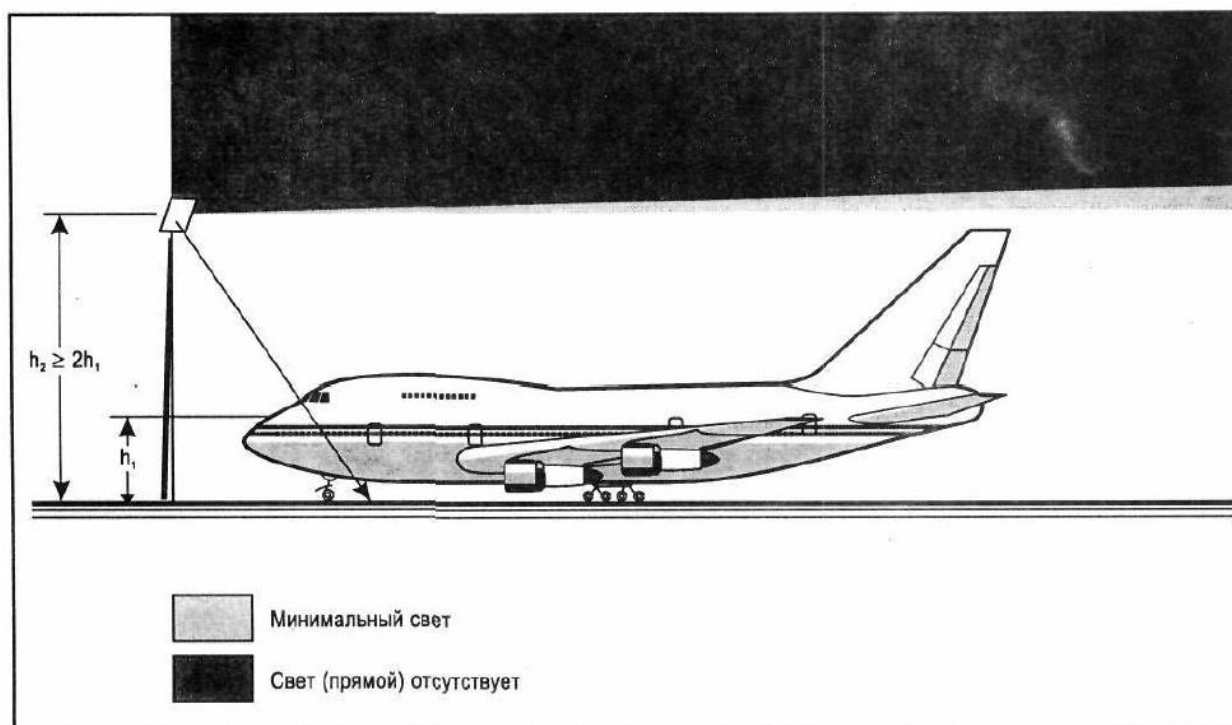
Рисунок 13-6. Установка по высоте, исключая блескость
