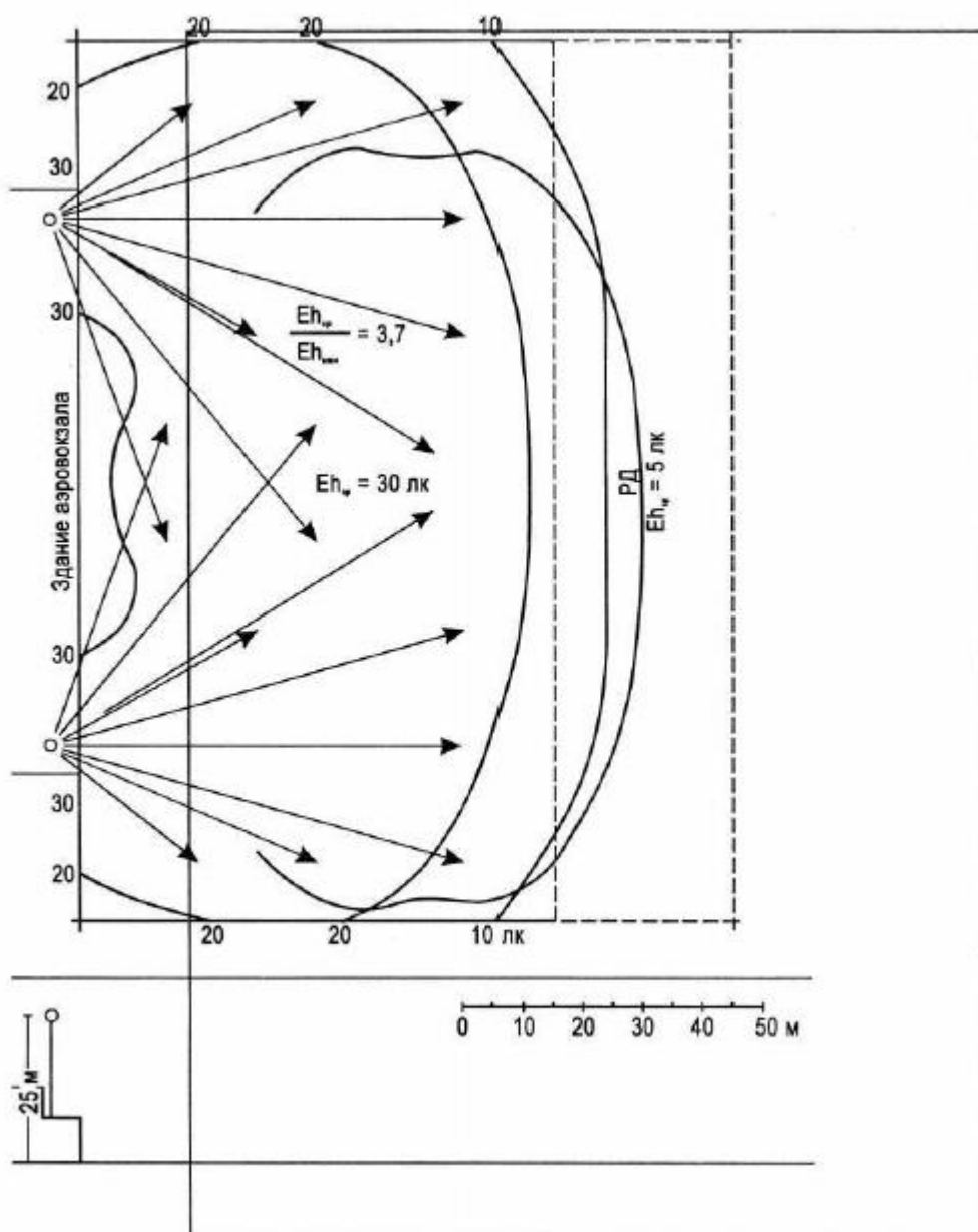
Рисунок 13-1. Типовые кривые равной освещенности в горизонтальной плоскости (пример А)
