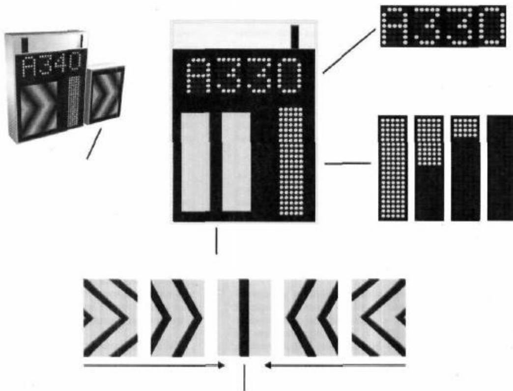
Рисунок 12-2. Система управления визуальной стыковкой воздушного судна с телескопическим трапом, в которой для указания азимутального направления используются графические табло с муаровым эффектом, а индикация располагаемой дистанции движения вперед и точки остановки осуществляется посредством лазерного локатора.
