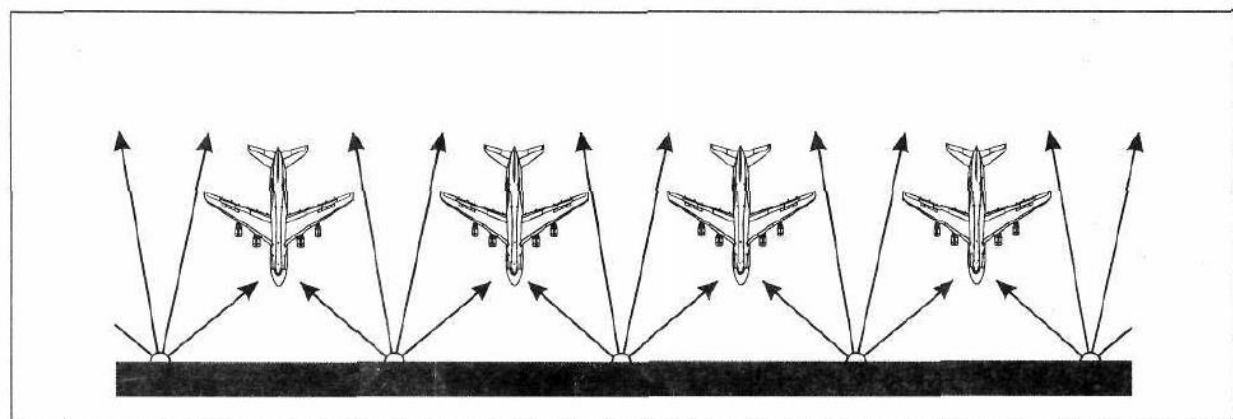
Рисунок 13-7. Типовая расстановка прожекторов и направление их лучей при параллельном размещении воздушных судов
