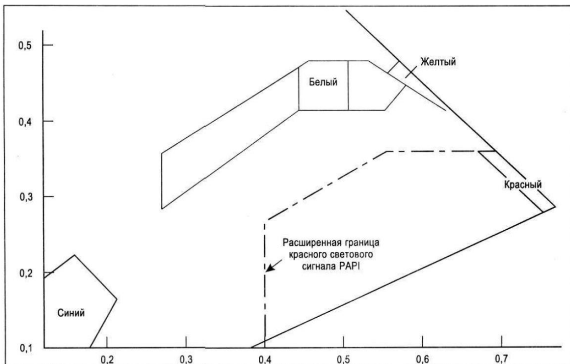
Рисунок 8-11. Предлагаемые целесообразные границы для красного светового сигнала РАРІ
