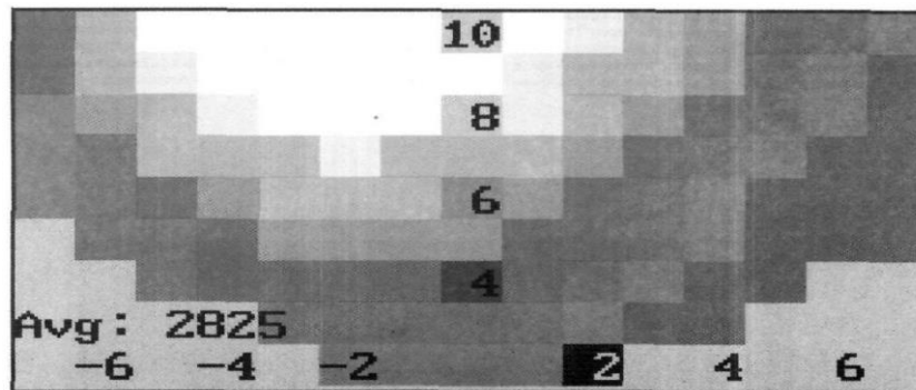
Рисунок 17-3А. Индикация данных контроля огня с нарушенной ориентировкой луча
