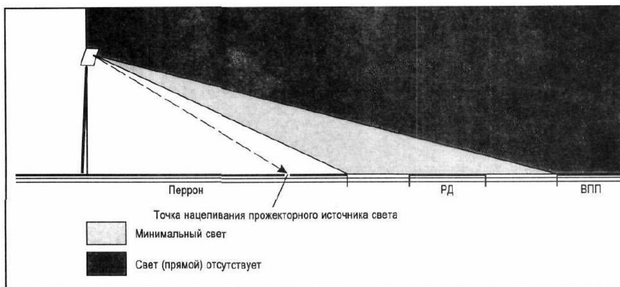
Рисунок 13-5. Нацеливание прожекторов для избежания блескости
