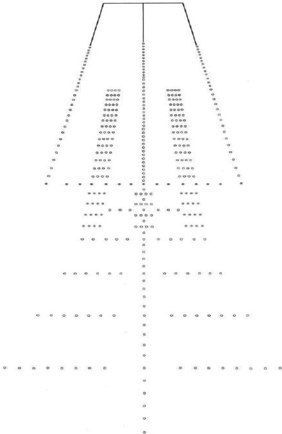
Рисунок 16-2. Системы огней приближения и освещения ВПП, сокращенная конфигурация
