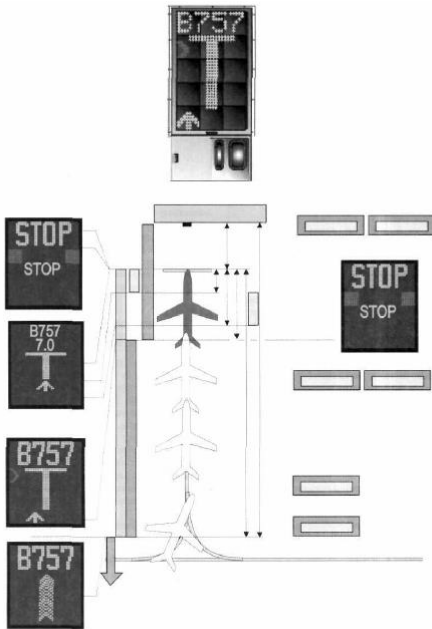
Рисунок 12-1. Система управления визуальной стыковкой воздушного судна с телескопическим трапом, в которой для индикации информации по азимутальному направлению, о располагаемой дистанции движения вперед и о требуемой точке остановки используются графические табло и лазерные датчики
