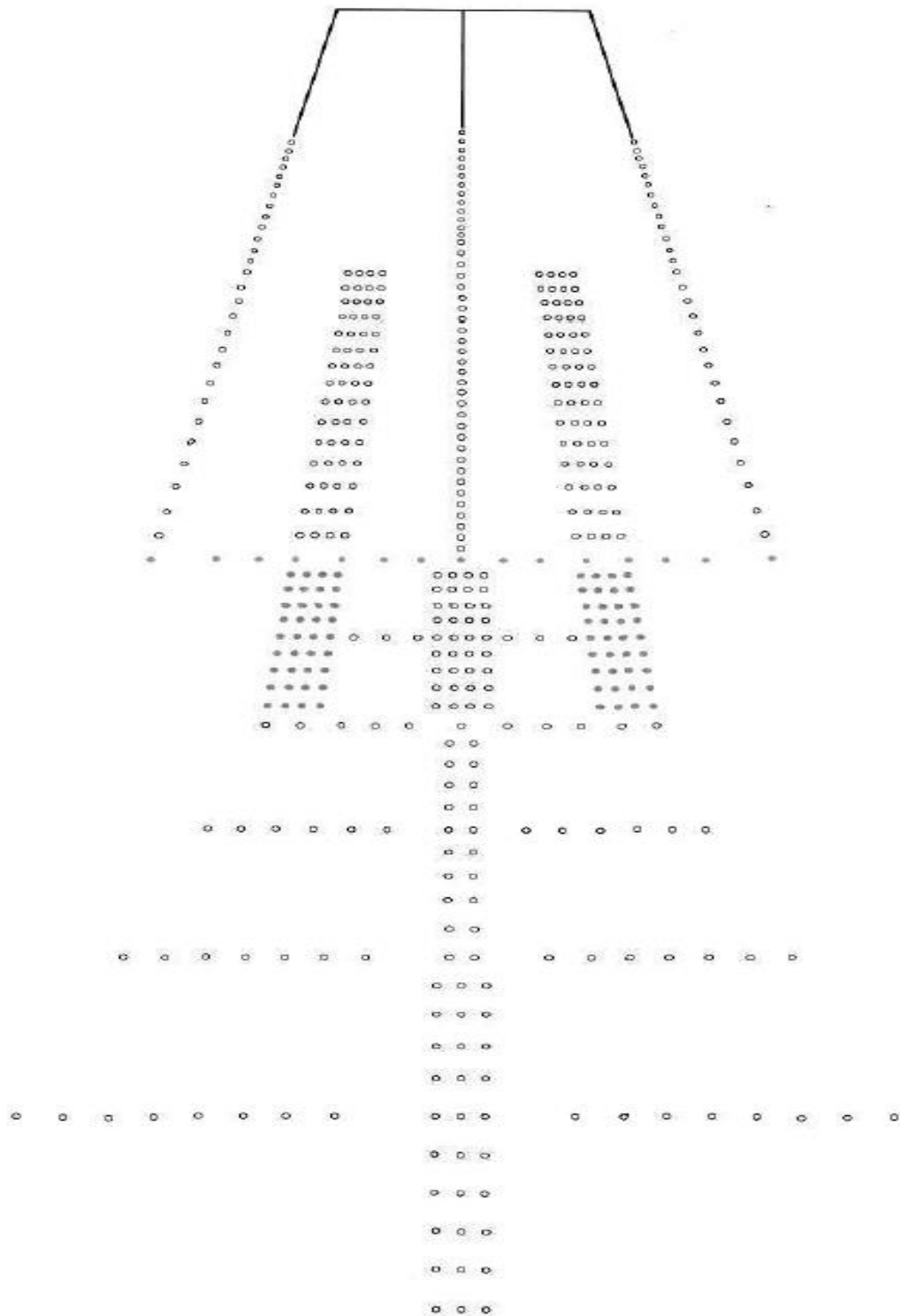
Рисунок 16-1. Системы огней приближения и освещения ВПП, полная конфигурация
