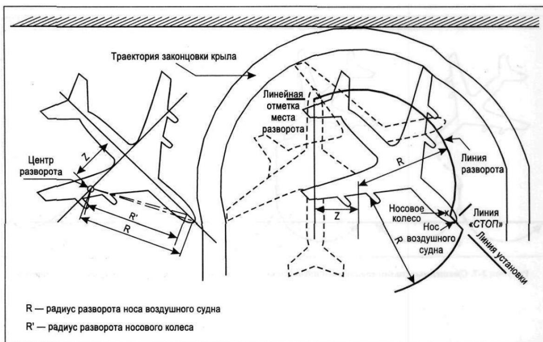
Рисунок 2-5. Линия разворота и контрольные отметки
