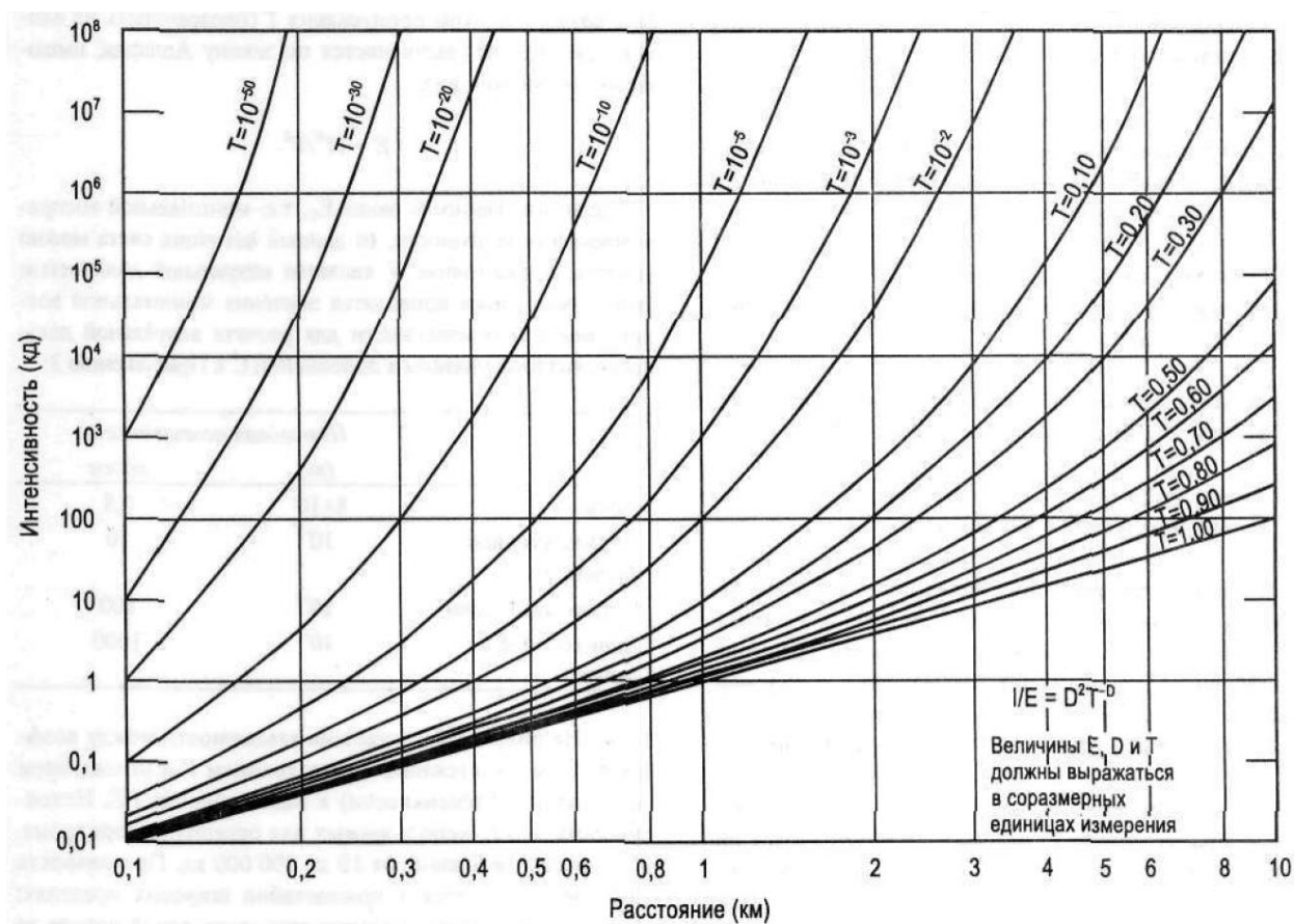
Рисунок 1-1. Интенсивность, необходимая для получения единичной освещенности, в зависимости от расстояния при различных коэффициентах пропускания атмосферы
