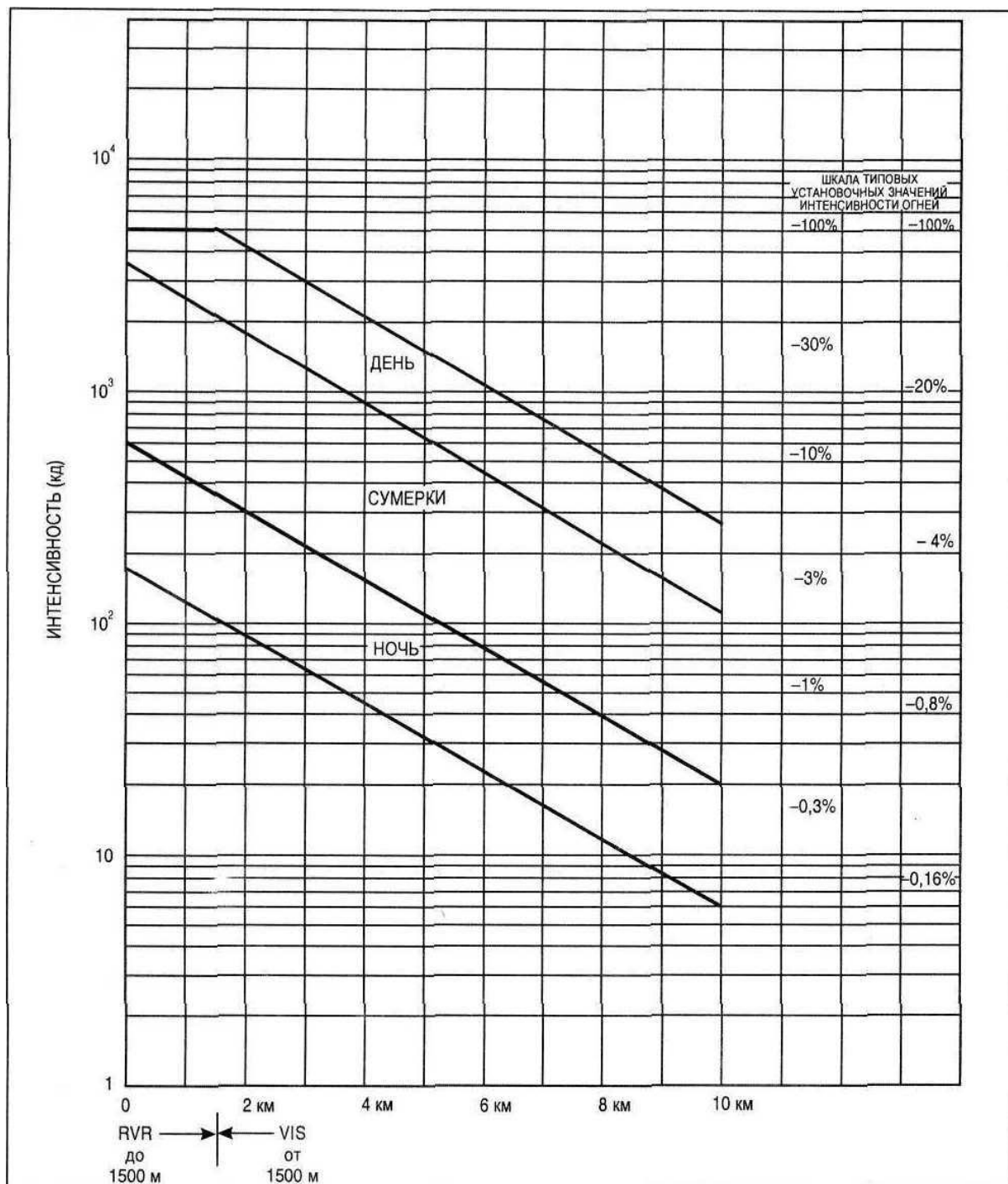
Рисунок 5-1. Центральный ряд огней приближения и световые горизонты
