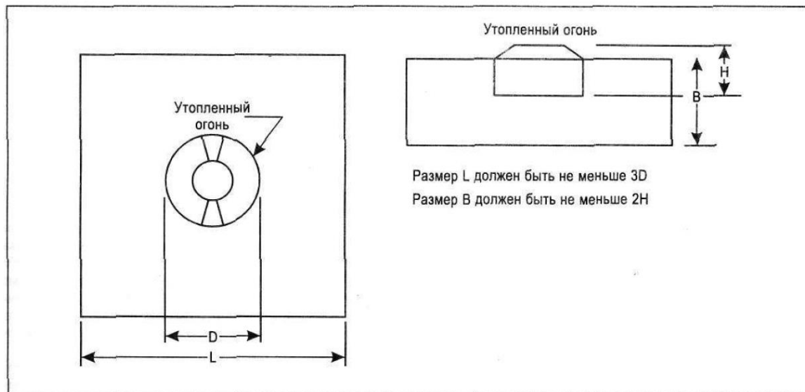
Рисунок 9-1. Типовой контейнер, используемый для измерения температуры утопленных огней
