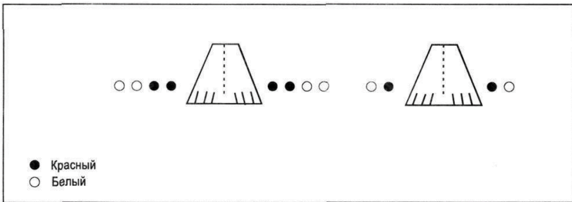
Рисунок 8-8. Огни PAPI и APAPI по обе стороны ВПП
