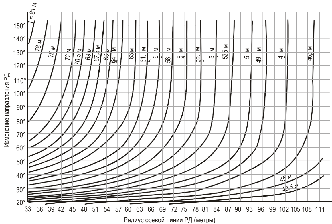
Рис. А1-20. Номограмма ускоренного расчета для Боинга-747 (кабина пилота над осевой линией РД)
