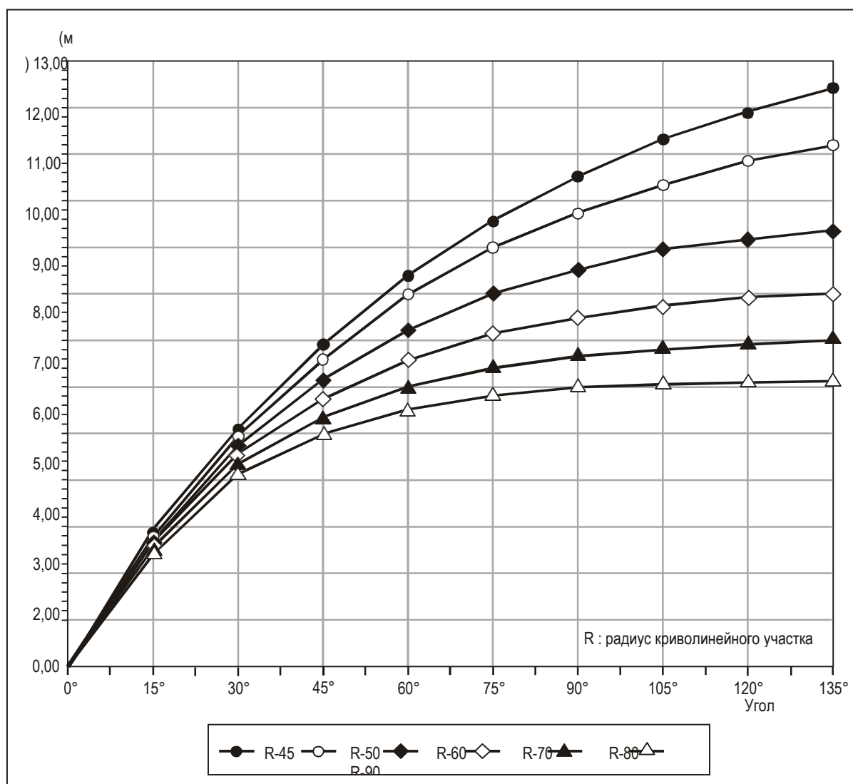
Рис. 1-7. Максимальная траектория движения законцовки крыла в зависимости от радиуса криволинейного участка "R" и угла поворота для В-777-300
