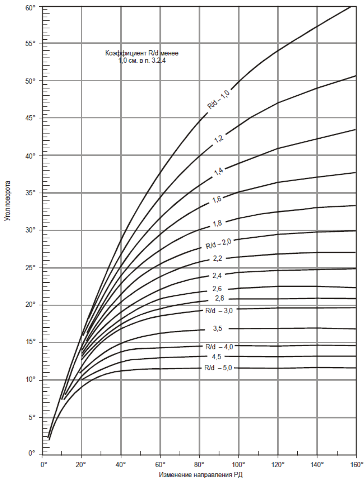
Рис. А1-16. Увеличение угла поворота при повороте
