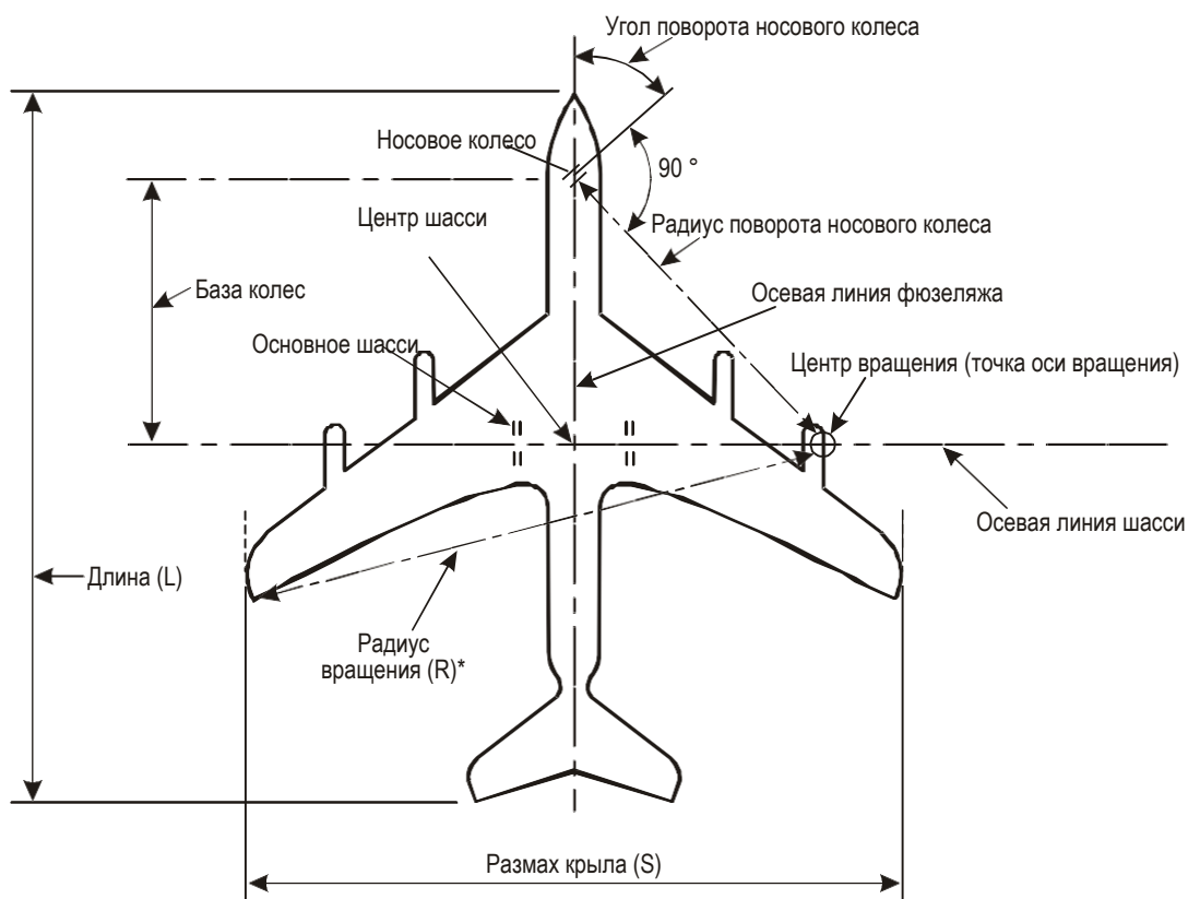
Рис. 3-3. Размеры для определения параметров места стоянки воздушного судна
