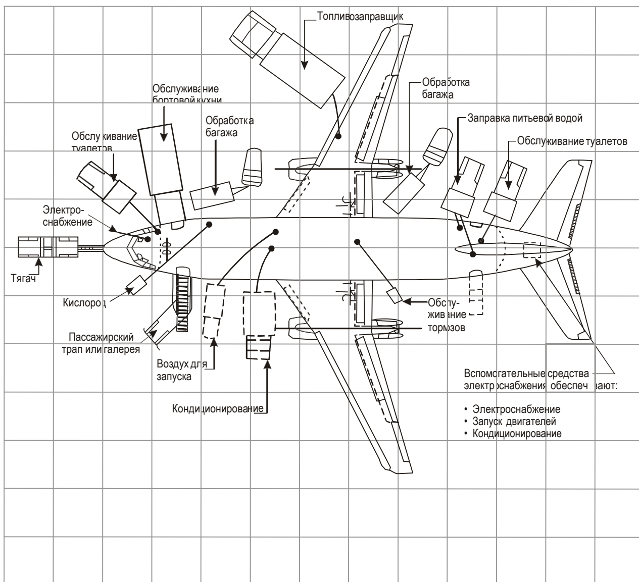
Рис. 3-5. Типовое размещение средств наземного обслуживания
