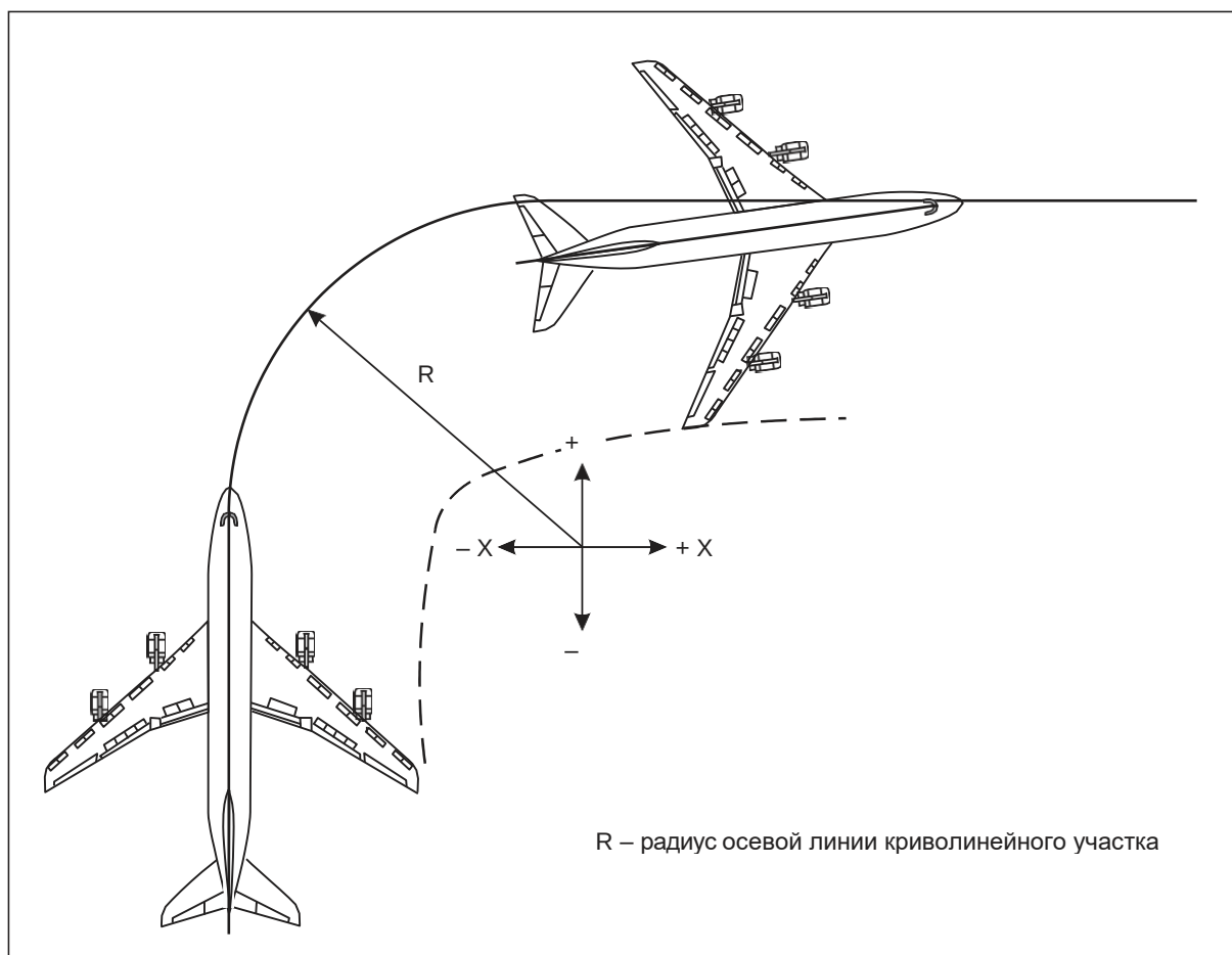
Рис. 1-6. Траектория движения законцовки внутреннего крыла (кабина экипажа над осевой линией РД)
