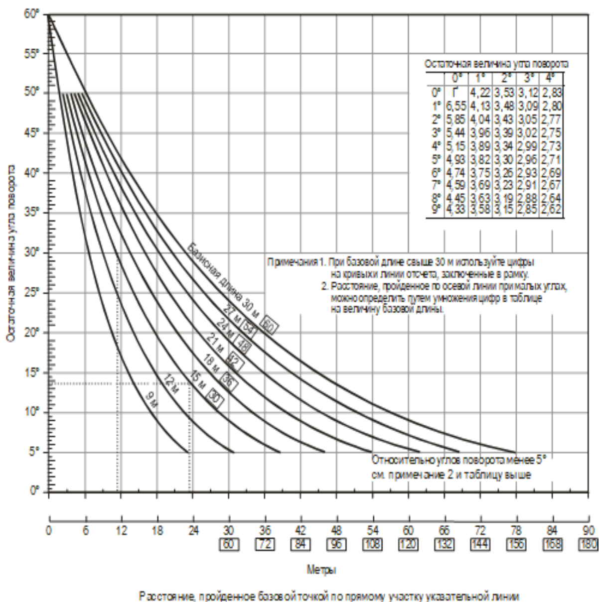
Рис. А1-17. Уменьшение угла поворота при завершении поворота
