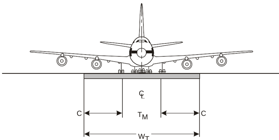
Рис. 1-18. Геометрическое построение ширины РД
