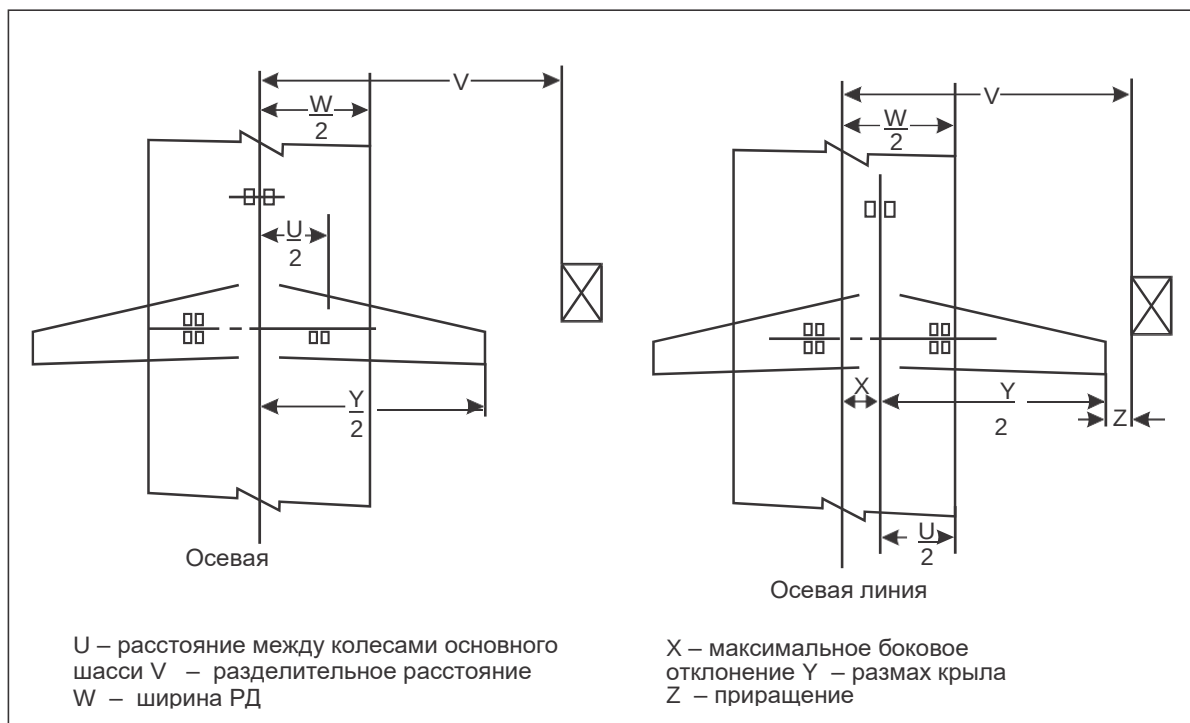
Рис. 1-4. Разделительное расстояние до объекта
