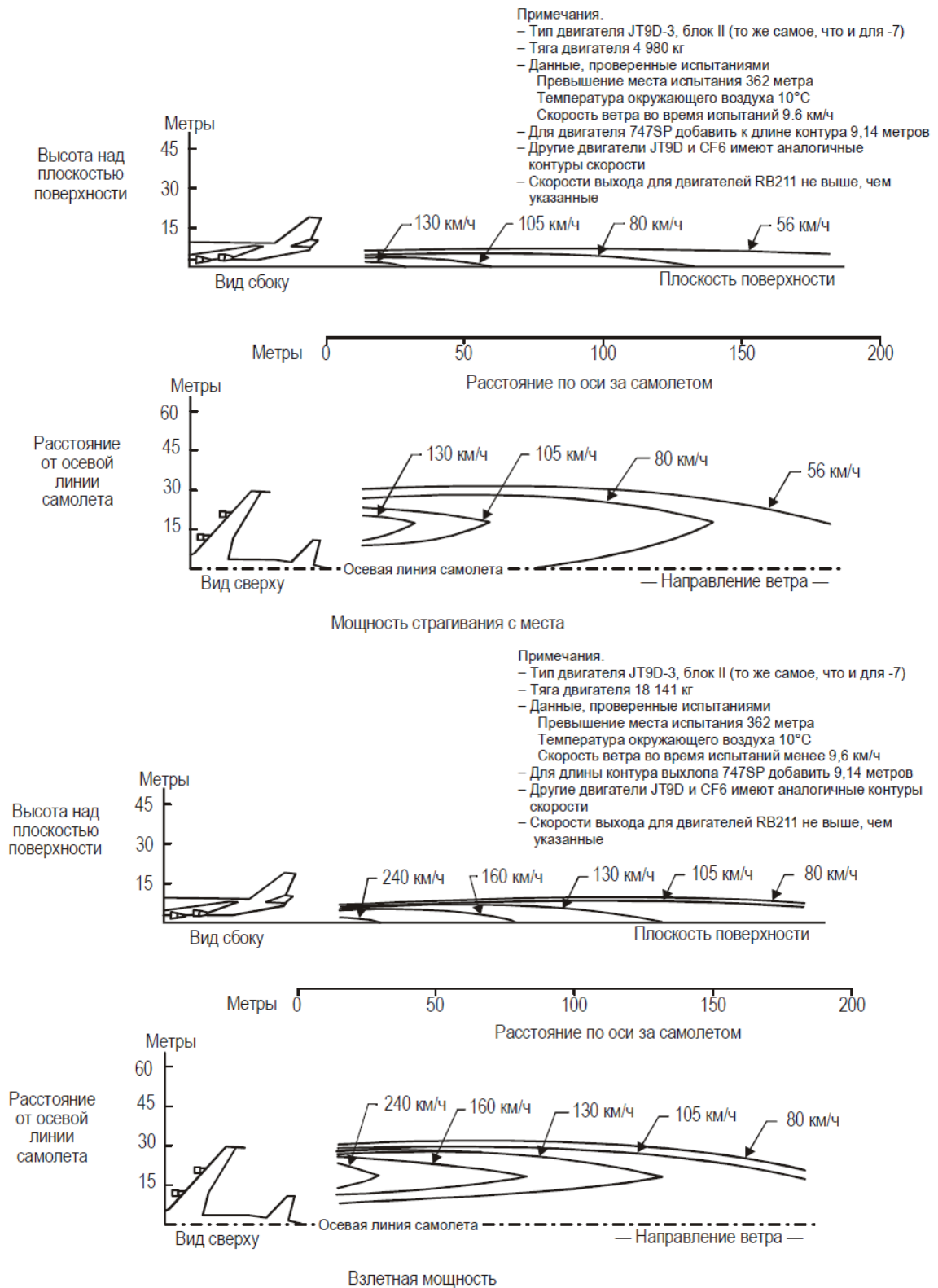
Рис. А2-7. Кривые зависимости скорости струи реактивного двигателя для самолета Боинг-747
