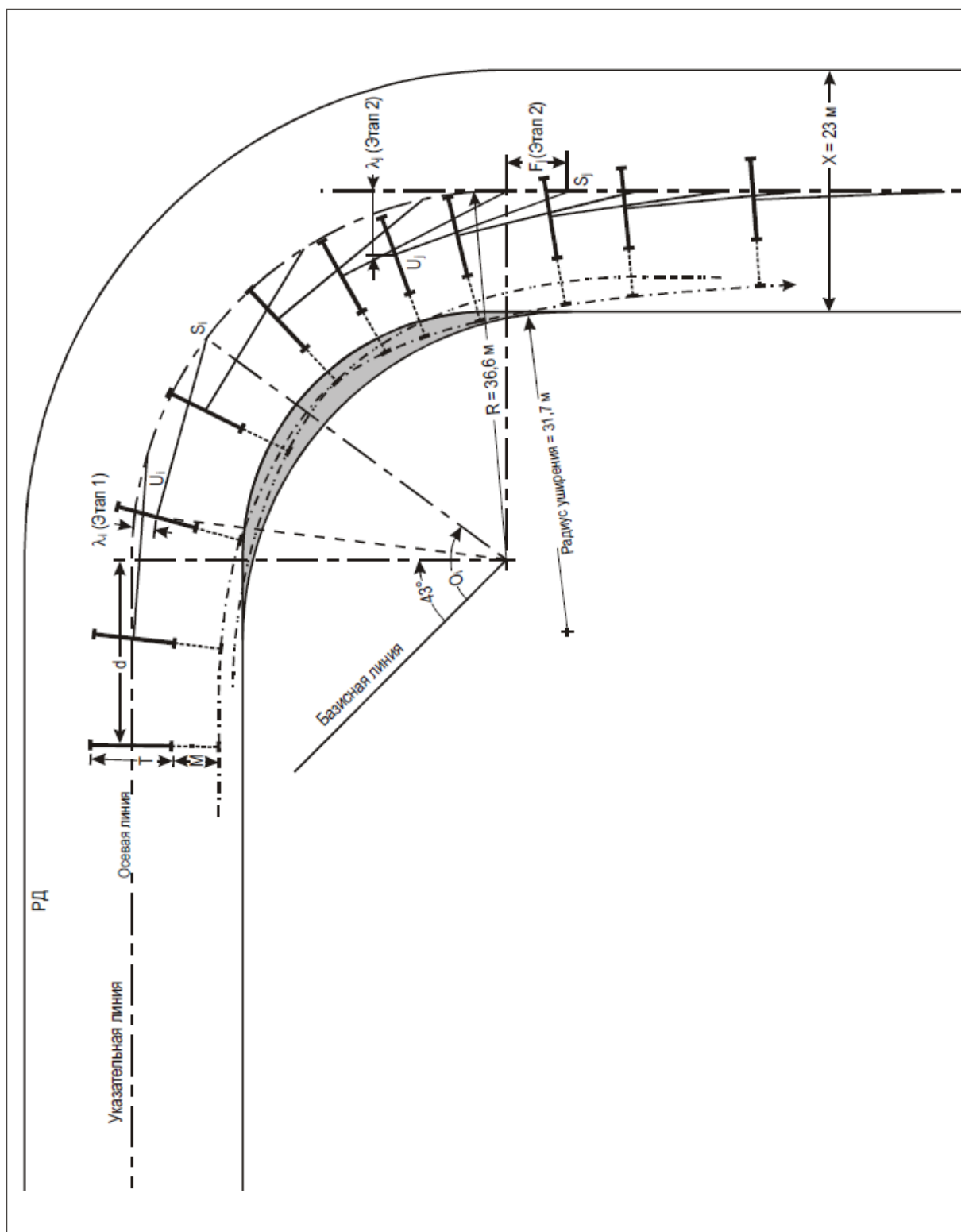
Рис. А1-12. Графический метод проектирования уширения
