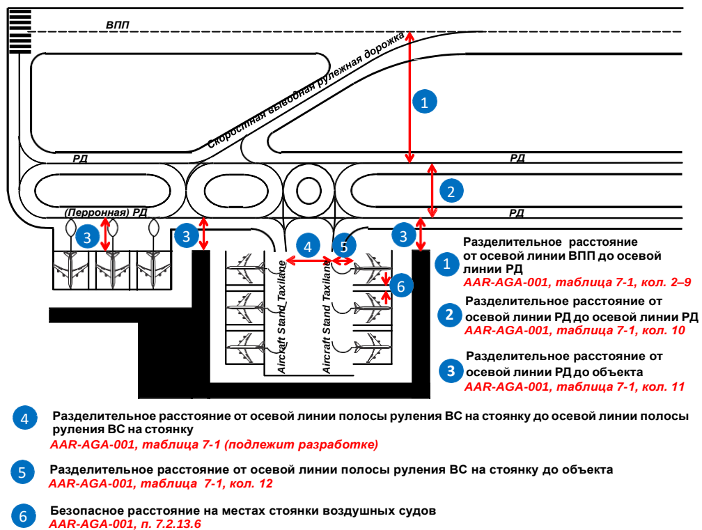
Рис. 1-2. Минимальные разделительные расстояния РД
