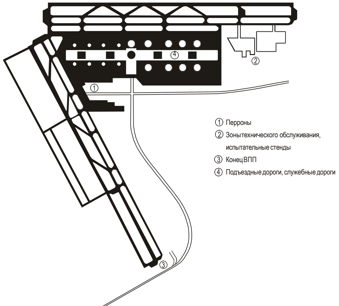
Рис. А2-10. Места на аэродроме, где необходимы струеотклоняющие щиты
