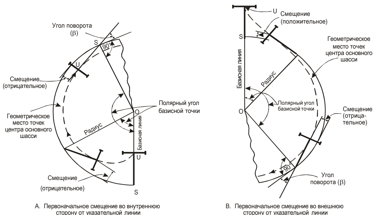
Рис. А1-5. Смещение центра основного шасси при следовании базисной точки по дуге окружности
