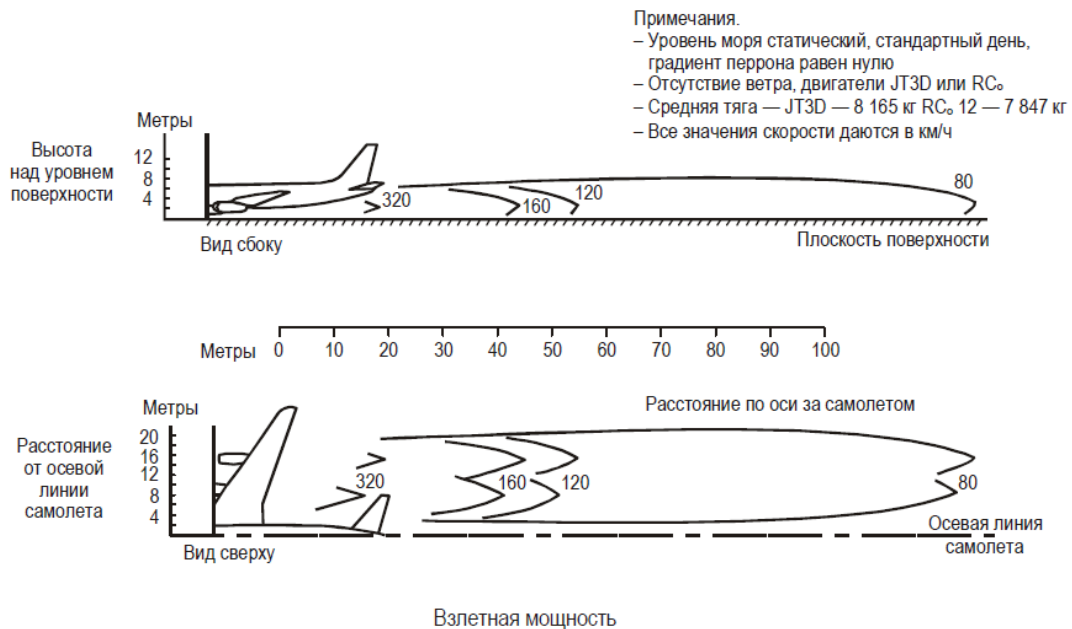
Рис. А2-5. Кривые зависимости скорости струи реактивного двигателя для самолета Дуглас DC-8
