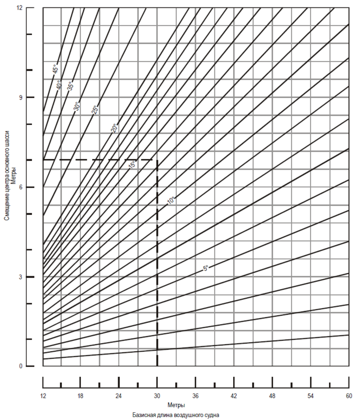
Рис. А1-15. Угол поворота ( \beta ) и смещение центра основного шасси ( \lambda ) (цифры на наклонных линиях обозначают величину угла поворота)
