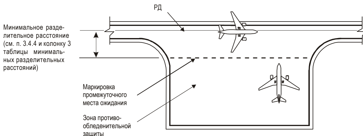
Рис. 3-6. Минимальное разделительное расстояние в зоне противообледенительной защиты
