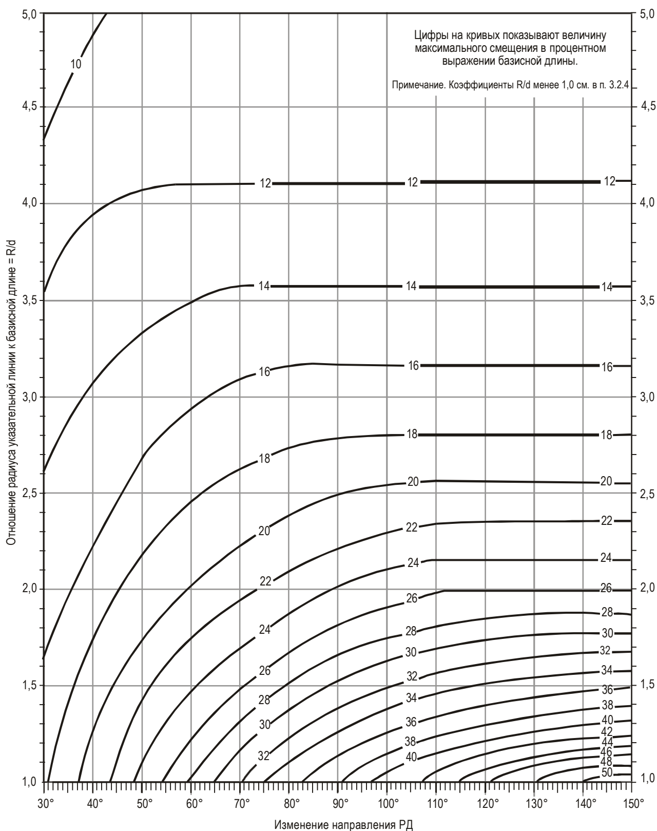
Рис. А1-14. Максимальное смещение ( \lambda_{\max} ) центра основного шасси
