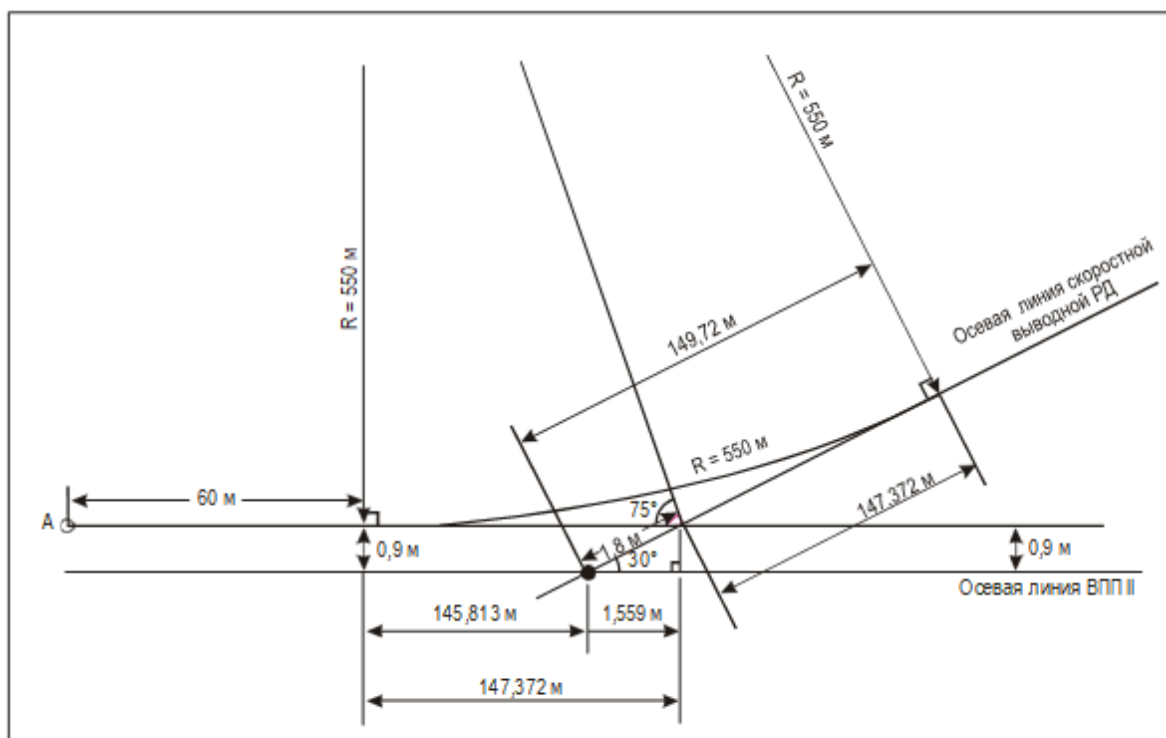
Рис. 1-14. Схема скоростных выводных РД (кодировый номер 3 или 4)
