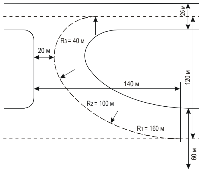
Рис. А5-3. Альтернативная схема выводной РД
