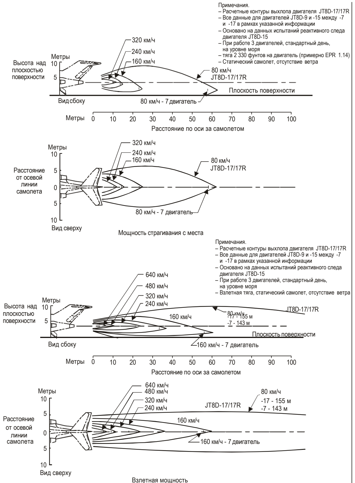
Рис. А2-6. Кривые зависимости скорости струи реактивного двигателя для самолета Боинг-727
