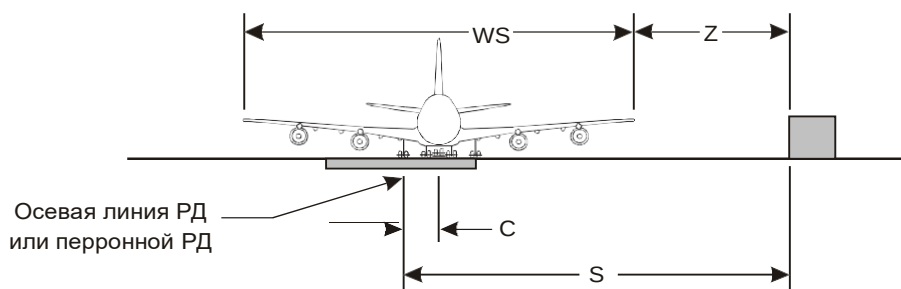
Рис. 1-21. Геометрическое построение расстояния от РД/ перронной РД до объекта
