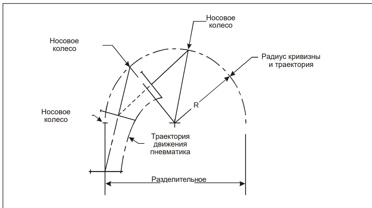
Рис. 1-5. Графическое решение разворота на 180°
