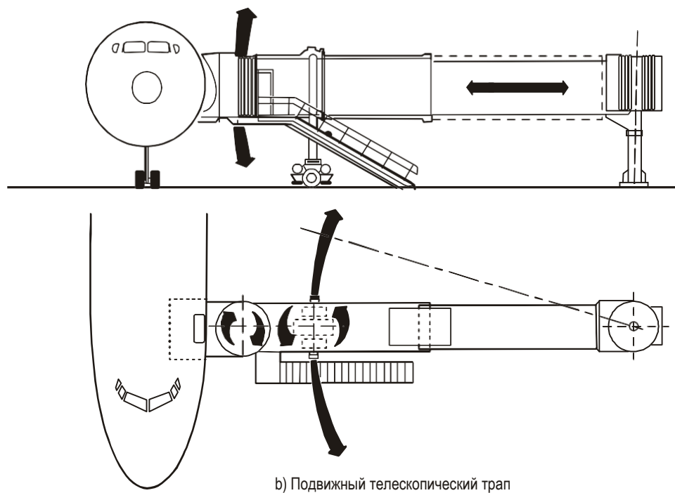
Рис. 3-1. Пассажирские телескопические трапы
