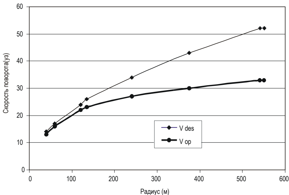
Рис. 1-16. Скорость воздушного судна в зависимости от радиуса скоростной выводной РД
