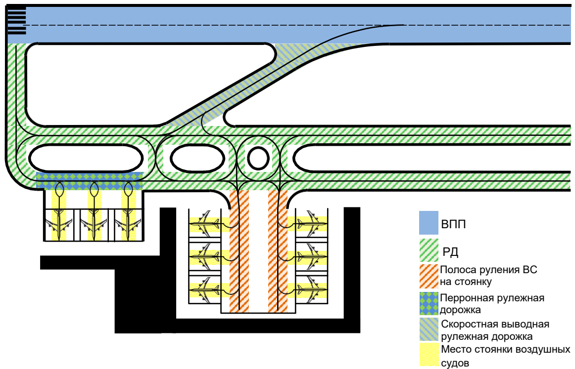
Рис. 1-1. Рулежные дорожки на перронах
