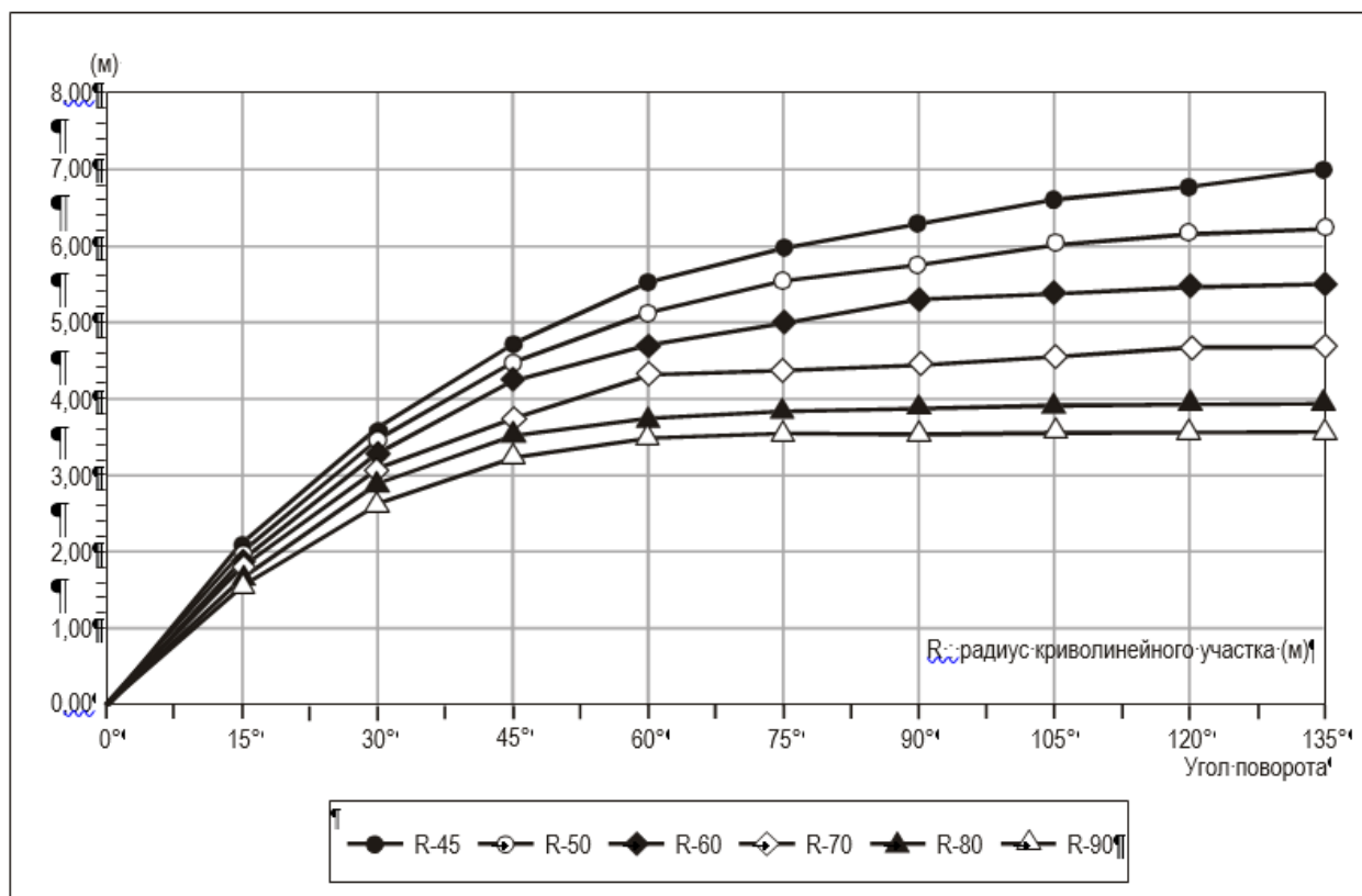
Рис. 1-9. Максимальная траектория движения законцовки крыла в зависимости от радиуса криволинейного участка "R" и угла поворота для В-747-400
