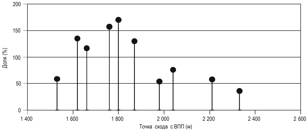
Рис. А5-2. Оптимальная точка схода с ВПП
