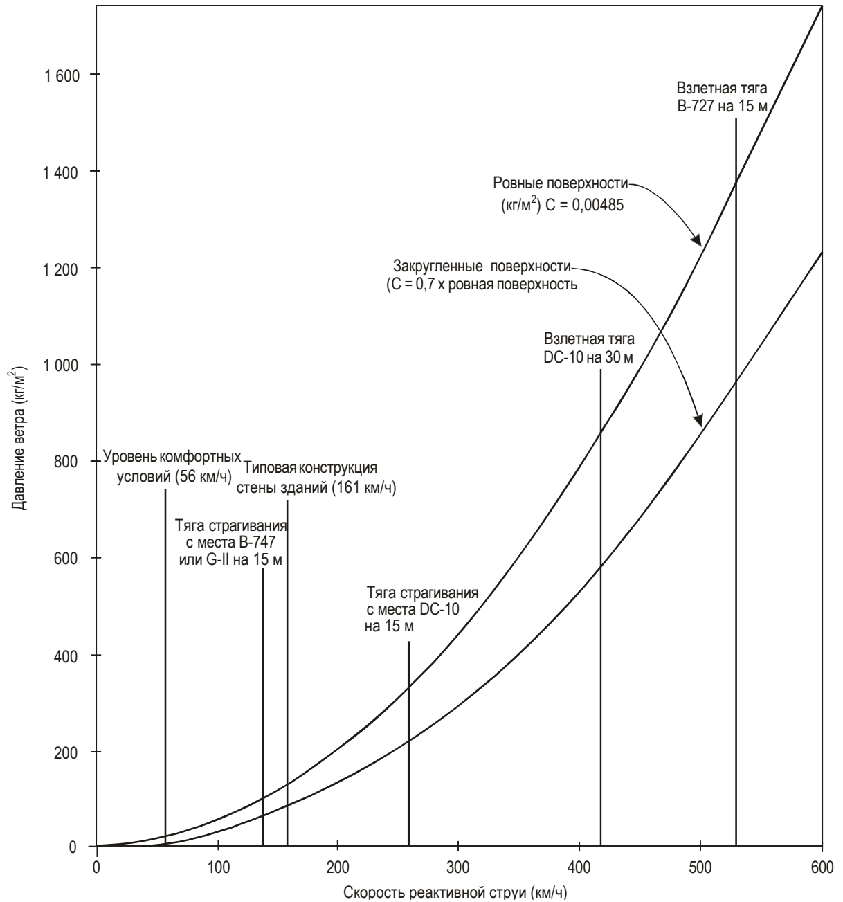
Рис. А2-9. Зависимость давления ветра от скорости реактивной струи
