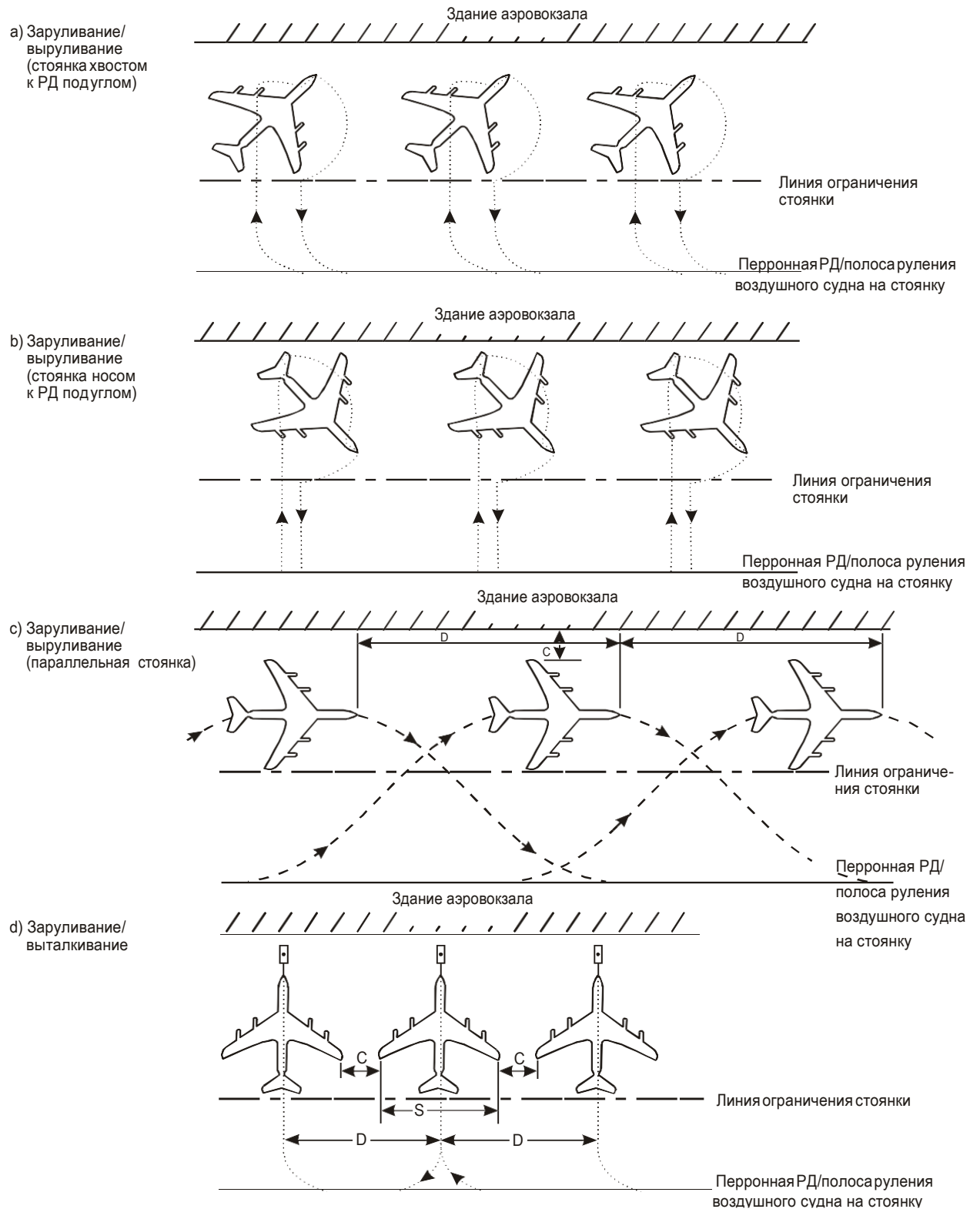
Рис. 3-4. Безопасная зона, необходимая для заруливания на место стоянки
