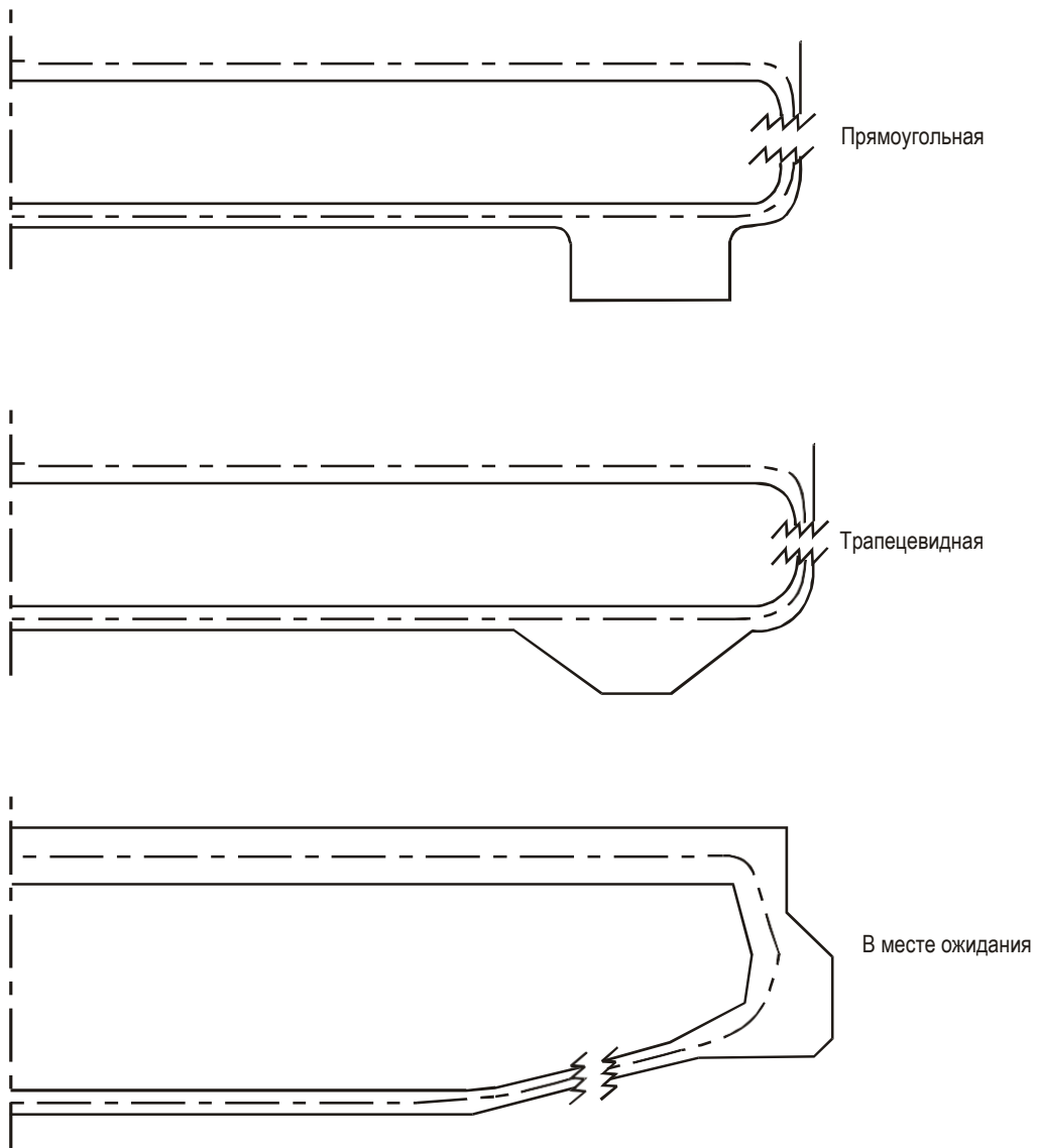
Рис. 2-1. Примеры схем площадок ожидания
