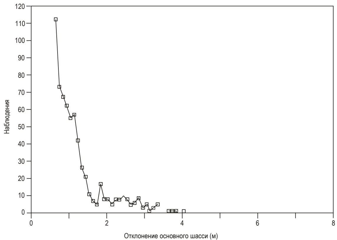
Рис. А4-1. Отклонения основного шасси В - 747 на прямолинейных участках РД
