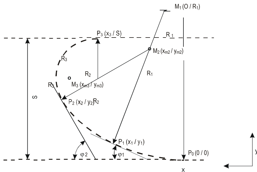
Рис. А5-4. Расчет кривой поворота
