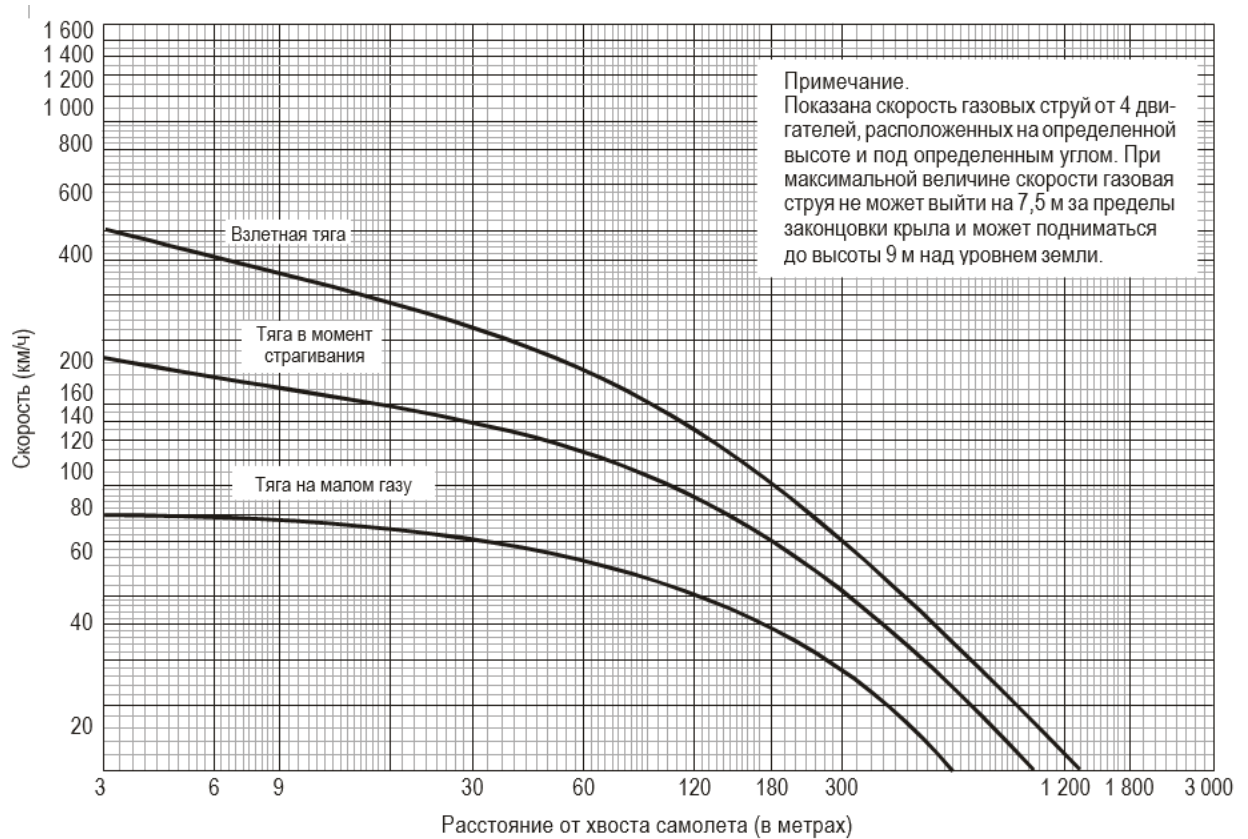
Рис. А2-3. Кривые максимальной скорости (В-747)
