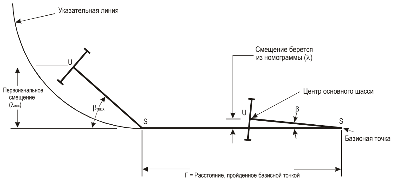
Рис. А1-6. Смещение центра основного шасси при следовании базисной точки по прямой линии
