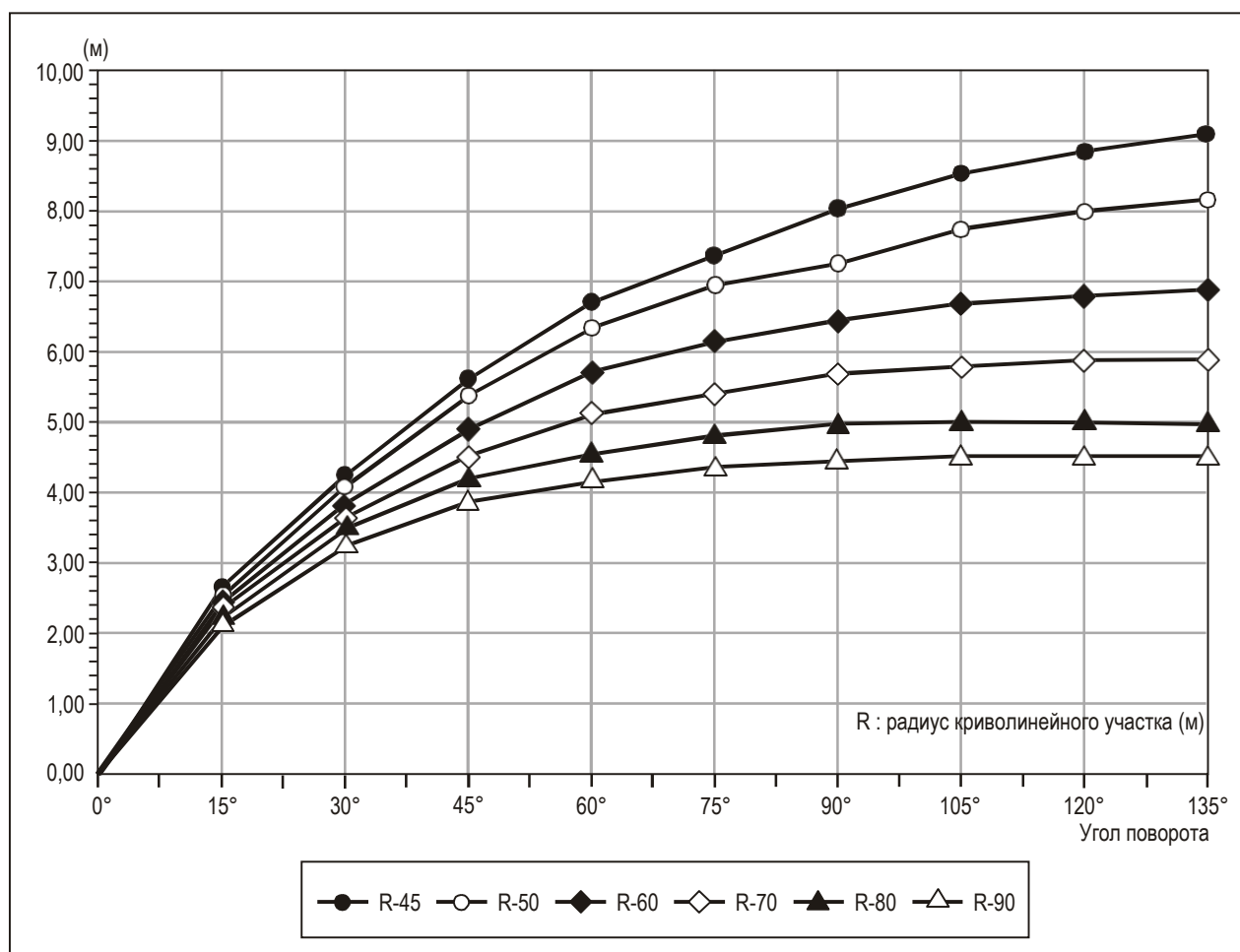
Рис. 1-11. Максимальная траектория движения законцовки крыла в зависимости от радиуса криволинейного участка "R" и угла поворота для А-330-300/А-340-300
