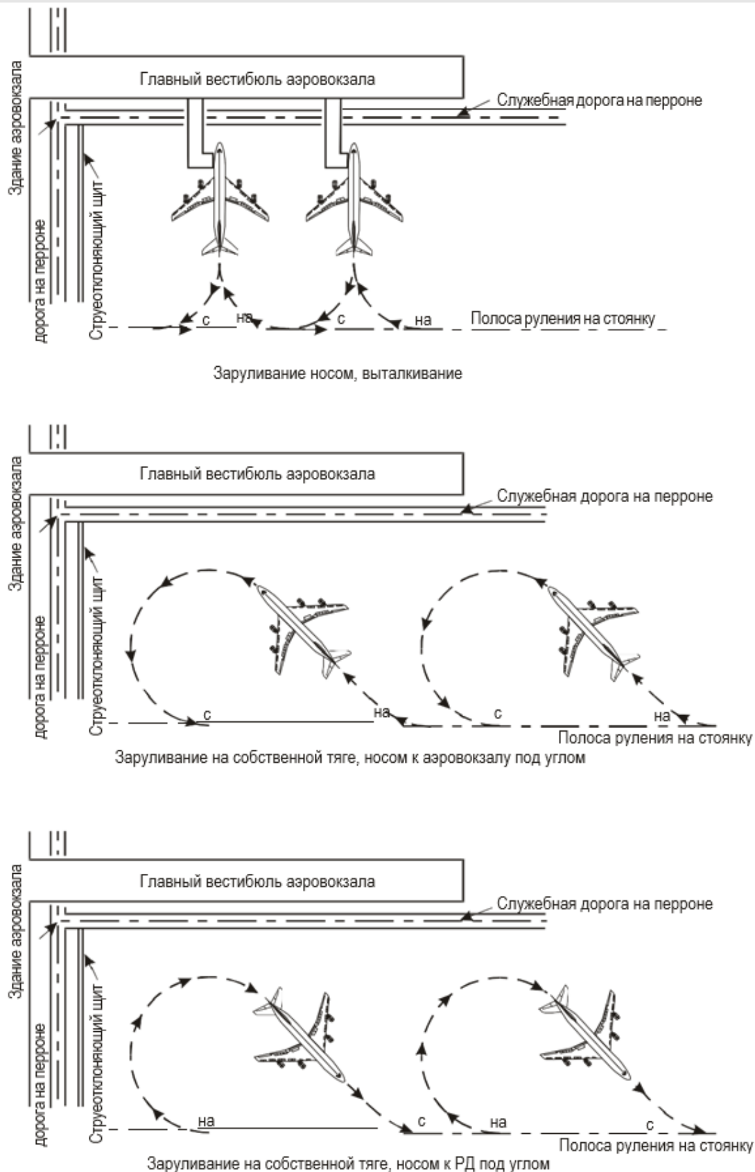
Рис. А2-11. Струеотклоняющие щиты в зонах перрона
