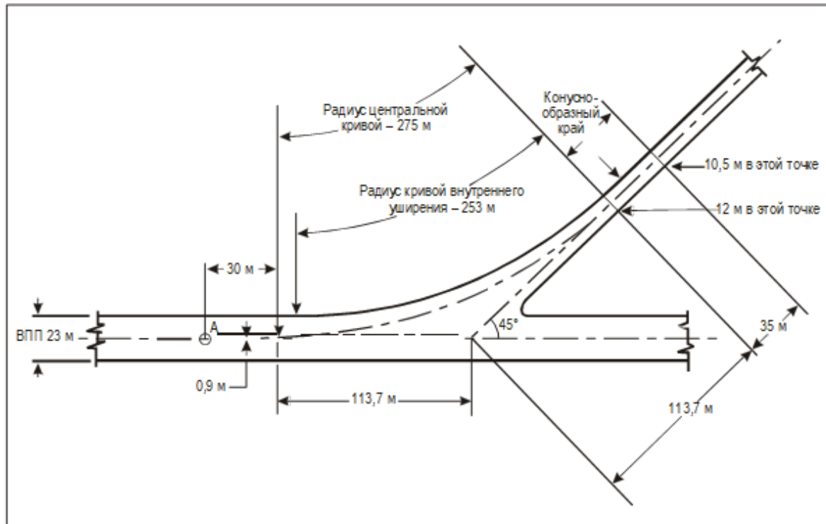
Рис. 1-13. Схема скоростных выводных РД (кодировый номер 1 или 2)
