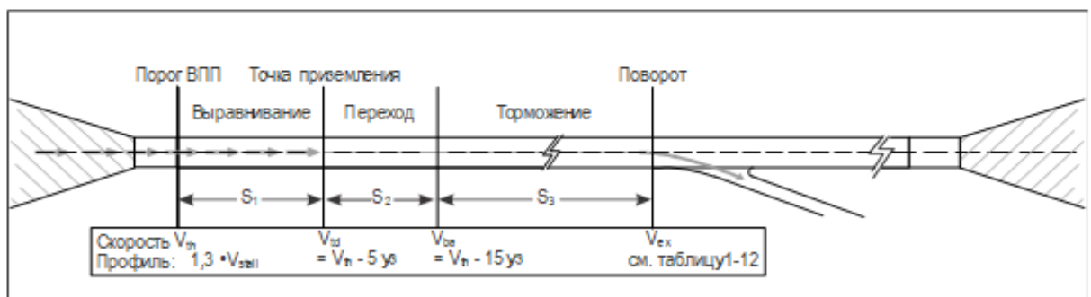
Рис. 1-15. Метод трех участков
