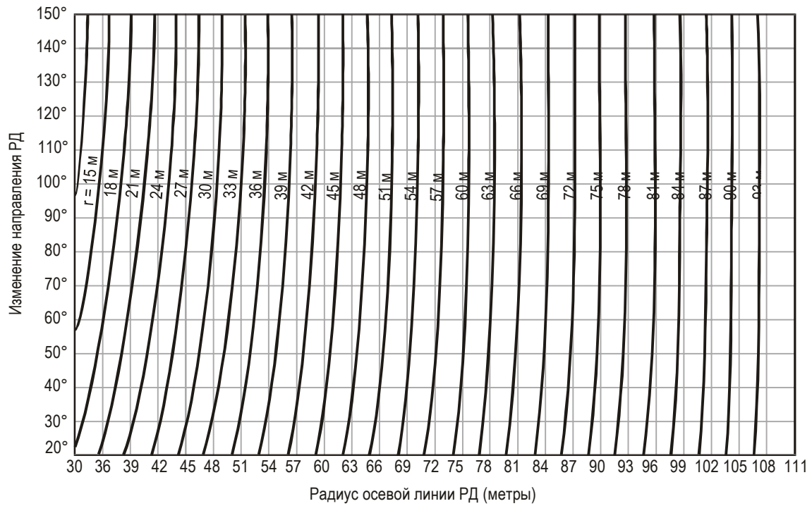
Номограмма А. Радиус дуги уширения (r)
