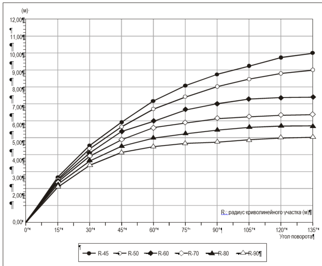
Рис. 1-8. Максимальная траектория движения законцовки крыла в зависимости от радиуса криволинейного участка "R" и угла поворота для MD-11
