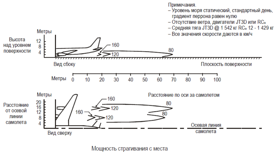
Рис. А2-4. Кривые максимальной скорости (DC-10)
