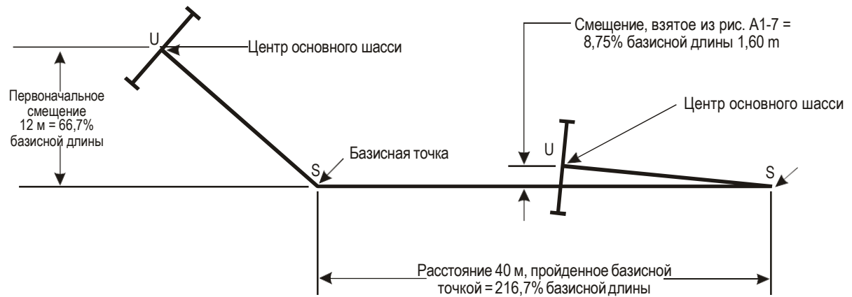
Рис. 1-8. Пример смещения центра основного шасси (U) при следовании базисной точки по прямой линии
