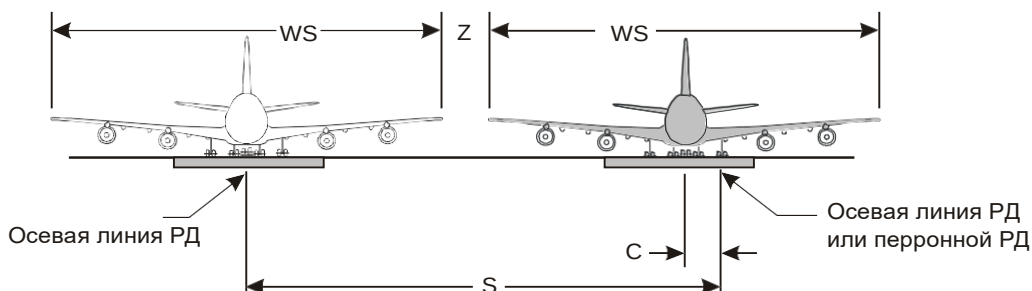
Рис. 1-20. Геометрическое построение разделения параллельных РД
